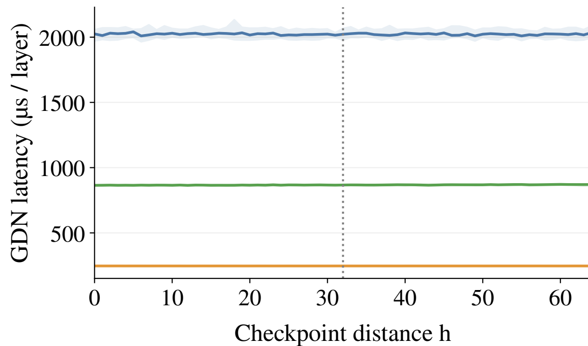
(d) Draft = 32
