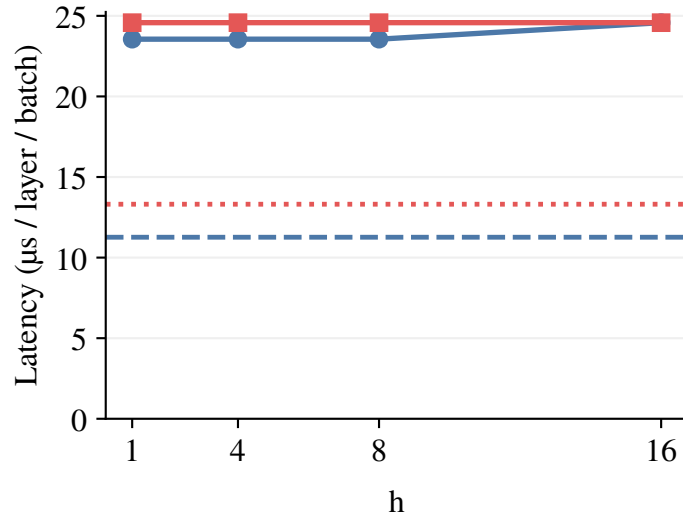
(b) bs=8
