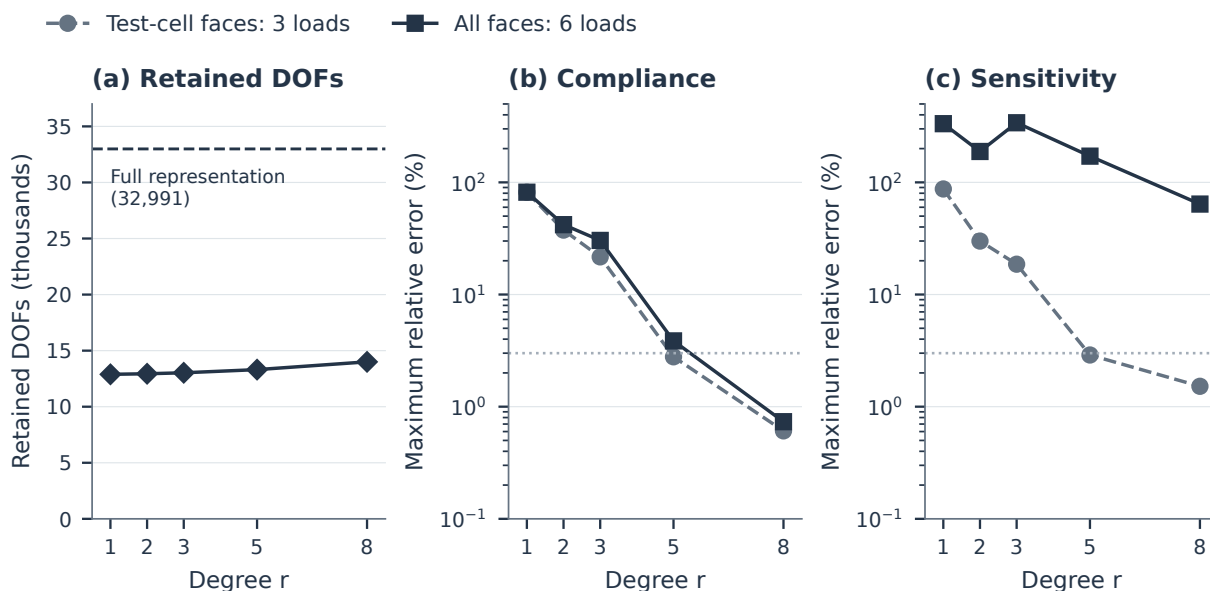
图 12: 限制胞元表面位移引起的响应误差。H1/x 的两个胞元均采用精确凝聚刚度矩阵，并在每个胞元表面上采用 r 次 Bernstein 多项式。切割平面单元中不在胞元表面上的自由度不受限制。(a) 主自由度数目；虚线表示完整表示的 32,991 个自由度。(b,c) 被测胞元表面三个载荷下或被测胞元与相邻胞元表面全部六个载荷下的最大柔度误差和最大被测胞元灵敏度误差。不计切割面上的面力载荷。误差以采用全部主自由度的解为基准，水平线标示 3%。
