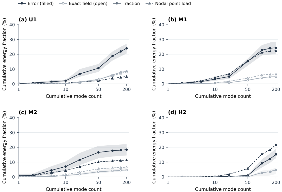
图 6: 基础网络内部位移误差的谱分布。各子图依次为 U1、M1、M2 和 H2。模式满足 Av = \lambda Dv ，其中 D = \text{diag}(A) ，并按特征值递增排序。深色实心标记表示误差，浅灰色空心标记表示精确内部位移场。带圆形标记的实线对应面力载荷，带三角形标记的虚线对应集中节点载荷。曲线为各测试位移的均值。色带为面力载荷下各测试位移的第 10 至第 90 百分位数。每条累积占比曲线均以其自身位移场或误差的内部总能量归一化。
