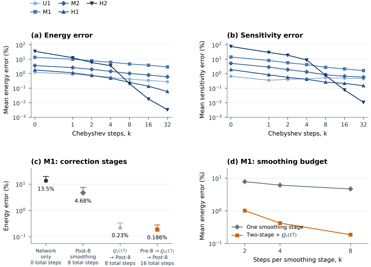
图 8: 固定网络参数下对基础网络的修正。(a,b) 五个胞元在 Chebyshev 光滑过程中的平均能量误差与灵敏度误差。(c) M1 在四种情形下的结果: 无修正; 八步光滑; 粗网格校正后接八步光滑; 粗网格校正前后各八步光滑。圆点表示均值, 端帽表示第 90 百分位数。(d) M1 的平均能量误差随每个光滑阶段步数 k 的变化, 分别对应单独一个光滑阶段, 以及由 k 步前光滑、 Q_1(17) 粗网格校正和 k 步后光滑组成的循环。所有子图均采用面力载荷、固定的主自由度位移和 a = b/30 。(a,b) 中步数轴在零到一之间为线性刻度, 此后为对数刻度。
