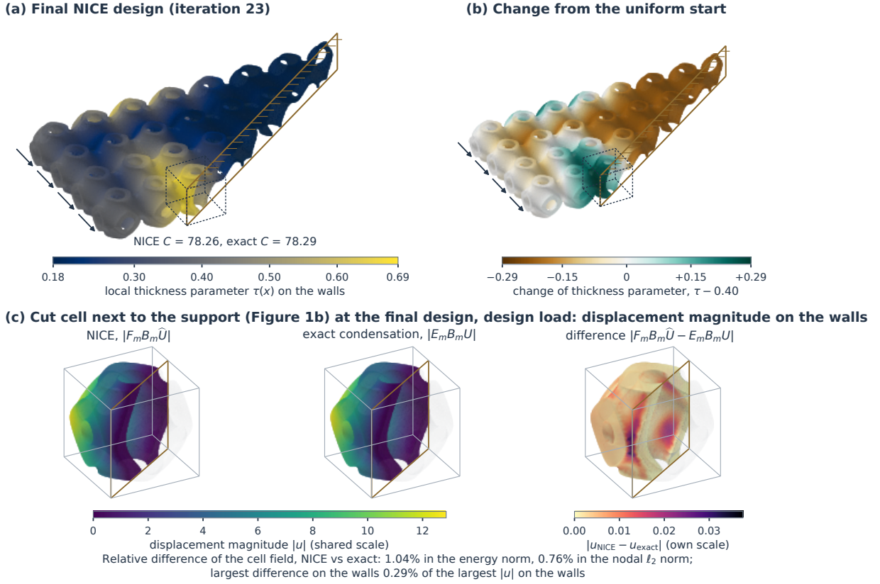
图 13: 切割面固支板的厚度设计。(a) NICE 最终设计，壁面按局部厚度参数着色，并标出 NICE 柔度与精确柔度（补充表 ST21）。(b) 相对均匀初始设计的变化 \tau - 0.40 。材料向加载端附近紧邻支撑的胞元集中（最多 +0.29），远离载荷的胞元则被减薄（最多 -0.22）。(c) 图 1b 中的切割胞元在最终设计和设计载荷下的位移。图中给出 NICE 恢复位移场 F_m B_m \hat{U} 与精确静力凝聚 E_m B_m U 在壁面上的位移大小，二者采用同一色标，二者之差采用单独的色标。两个位移场在该胞元能量范数下相差 1.04%，在节点位移欧氏范数下相差 0.76%。将同一位移恢复算子作用于精确的主自由度位移，同样得到 1.04%，因此该差异来自胞元内部的位移恢复。在整块板上，能量范数下的差异为 1.72%，其平方等于柔度的相对差 2.96 \times 10^{-4} （式 (14)）。
