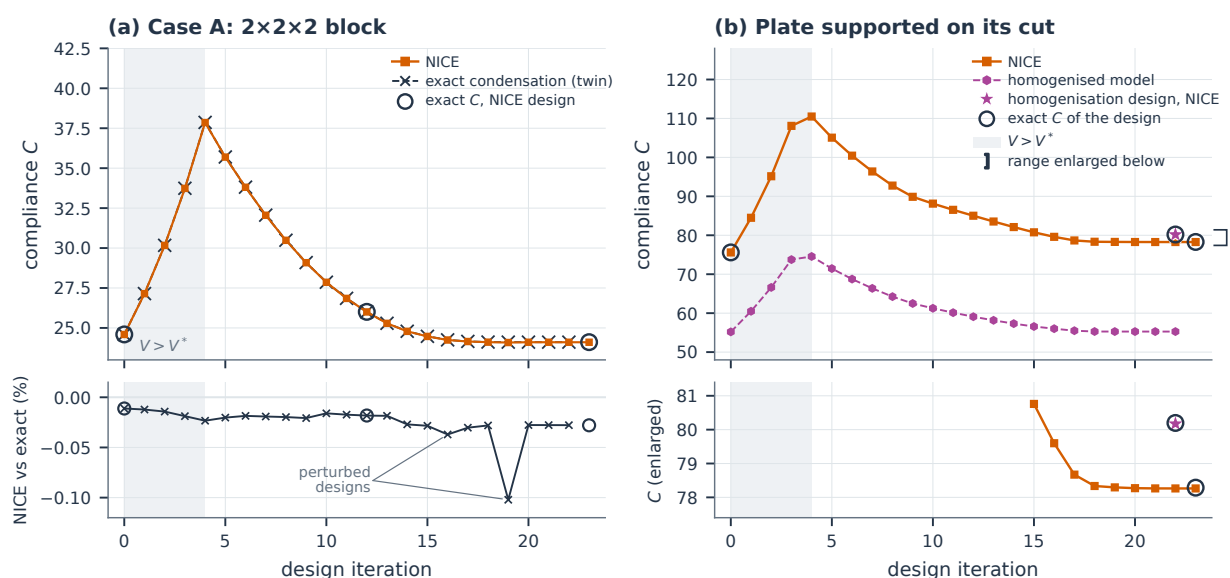
图 14: 基于 NICE 的厚度优化。(a) 算例 A: NICE 优化与采用精确静力凝聚的孪生优化的柔度历程。空心圆为 NICE 设计在第 0、12 和 23 次迭代时的精确柔度。在体积由 1.25V^* 减小至 V^* 的过程中, 柔度先上升 (阴影, 第 0-3 次迭代)。下方条带: NICE 柔度相对于同一设计迭代处孪生运行柔度的偏差 (线), 以及相对于同一设计精确柔度的偏差 (圆: -0.011\% 、 -0.018\% 、 -0.028\% )。两次运行的设计在第 0-4 次迭代时重合, 此后不同。在第 16 和 19 次迭代 (图中标注为 'perturbed designs'), NICE 设计曾被几何生成器的回退机制扰动 (补充表 ST19a)。(b) 切割面固支板。曲线为从均匀初始设计出发的 NICE 柔度, 以及均匀化宏观模型沿其自身优化路径的柔度 (虚线)。星号表示在切割几何上用 NICE 分析的均匀化设计, 位于最后一次宏观迭代处。空心圆为均匀初始设计、最终 NICE 设计和均匀化设计的精确柔度。阴影: V > V^* 的设计迭代。下方条带: 括号所标范围的放大, 自第 15 次迭代起。
