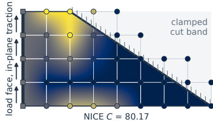
(b) Homogenisation design
