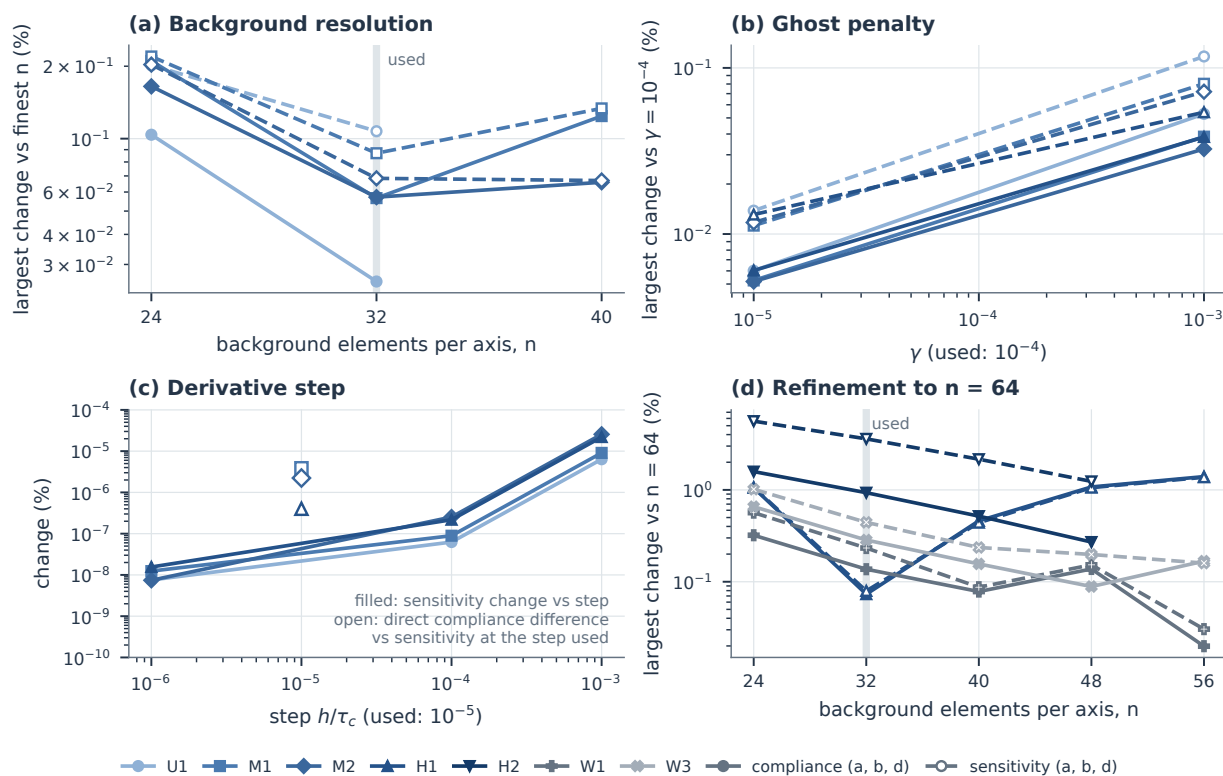
图 S01: CutFEM 参考解的验证。单个胞在一个盒面上固支，并在另一个面上沿三个笛卡尔方向分别受单位一致面力作用。在 (a)、(b) 和 (d) 中，带实心标记的实线表示柔度，带空心标记的虚线表示厚度灵敏度，均取三个载荷下的最大相对变化。(a) 相对于所计算的最细背景分辨率的变化，U1 为 n = 40 ，M1 和 M2 为 n = 48 ；全文所用参考解取 n = 32 。(b) ghost 罚项系数偏离全文所用值 10^{-4} 时的变化。(c) 实心：矩导数的有限差分步长偏离全文所用值 h_c = 10^{-5}\tau_c 时灵敏度的最大相对变化，在 10^{-3}\tau_c 处至多为 2.6 \times 10^{-5}\% ，在 10^{-4}\tau_c 处再小一百倍；空心：在所用步长下，柔度中心差分与灵敏度之间的最大相对差异。(d) H1、H2 以及 NICE 误差最大 (W1) 和壁厚最薄 (W3) 的验证胞加密至 n = 64 ，数据见表 ST10；H2 没有 n = 56 的解。
