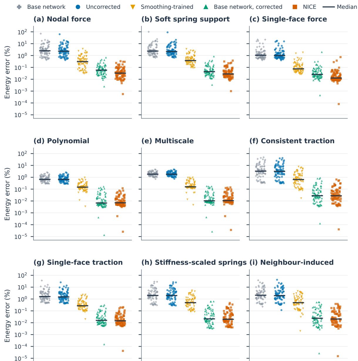
图 S02: 几何层面方向能量误差的分布。每个点表示一个验证几何在恒等取向下的平均方向能量误差；水平短线为总体中位数。节点力、弹簧支撑、单面力、多项式、多尺度、一致面力和单面一致面力各类包含 80 个几何，刚度缩放支撑和邻胞诱导位移两类各包含 75 个，与表 ST03 的总体相同。表 ST03 的五种变体（基础网络、未校正、平滑训练、部署时施加校正的基础网络、NICE）采用与正文图中相同的标记和颜色；以确定性的水平偏移区分重叠的观测点。所有子图共用对数误差轴。
