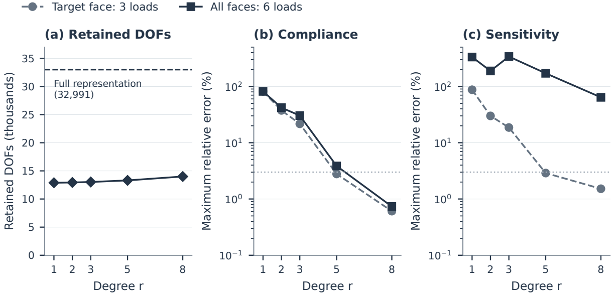
图 11: 限制盒面位移引起的响应误差。H1/x 的两个胞均采用精确算子, 并在每个盒面上采用 r 次 Bernstein 多项式, 非盒面切割带自由度不受限制。(a) 保留自由度数目; 虚线表示完整表示的 32,991 个自由度。(b,c) 在三个目标面载荷或全部六个目标面与邻胞面载荷下的最大柔度误差和最大目标胞灵敏度误差; 不计切割面内力。误差相对于完整保留空间解计算; 水平线标示 3%。
