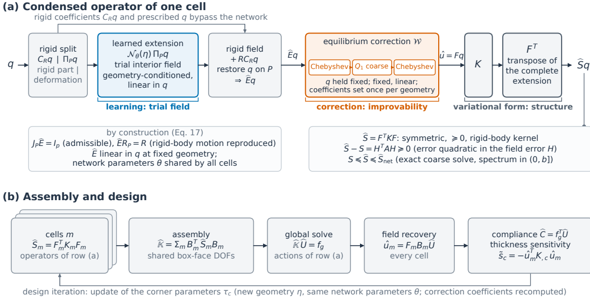
图 2: 学习位移延拓、平衡校正与变分装配。(a) 在由网络延拓变形之前，先从保留位移中分离出刚体运动。随后重构刚体场并恢复给定的保留值；校正 \mathcal{W} 接着在固定保留位移下减小内部不平衡，再施加局部刚度和完整延拓的转置 F^T ，即得到功共轭的保留力。(a) 中的排序假设粗求解精确或带非负平移，且光滑区间的上端界定谱；它对能量误差排序，而非对灵敏度误差排序。(b) 各胞算子在共享盒面自由度上装配，并求解装配系统；装配解为局部场恢复、柔度和场基厚度灵敏度提供输入。一次设计迭代更新角点厚度参数，从而重新生成每个胞的几何；网络参数保持不变，而 \mathcal{W} 的系数则重新计算。
