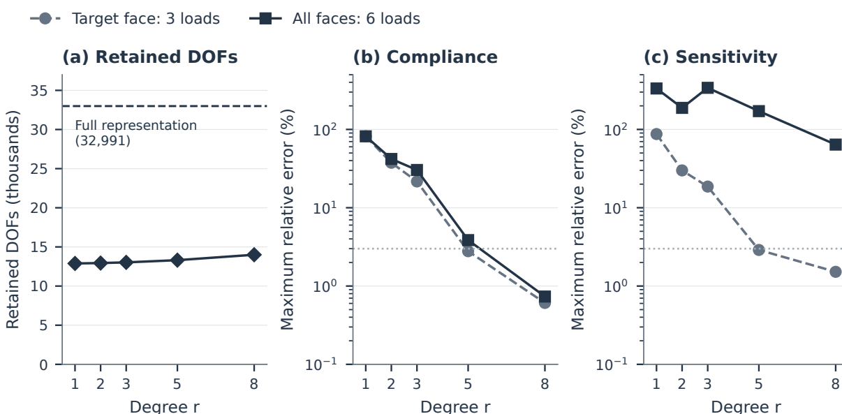
图 12: 限制胞元边界面位移引起的响应误差。H1/x 的两个胞元均采用精确算子，并在每个胞元边界面上采用 r 次 Bernstein 多项式，非胞元边界面切割带自由度不受限制。(a) 保留自由度数目；虚线表示完整表示的 32,991 个自由度。(b,c) 在三个目标面载荷或全部六个目标面与邻胞元面载荷下的最大柔度误差和最大目标胞元灵敏度误差；不计切割面面力。误差相对于完整保留空间解计算；水平线标示 3%。
