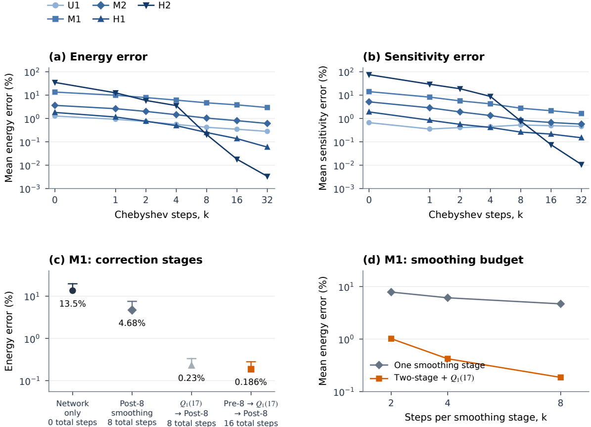
图 8: 在固定网络参数下校正基础网络所获得的精度提升。(a,b) 五个胞元上 Chebyshev 光滑过程中的平均方向能量误差与场基灵敏度误差。(c) M1 在以下情形下的结果：无校正、八步光滑、粗网格校正后接八步光滑，以及粗网格校正前后各八步光滑；圆点表示平均值，端帽表示第 90 百分位数。(d) M1：平均能量误差随每个光滑阶段步数 k 的变化，分别对应单独一个光滑阶段，以及 k 步前光滑、 Q_1(17) 粗网格校正与 k 步后光滑的组合。所有子图均采用一致面力、固定保留位移以及 a = b/30 ；在 (a,b) 中，步数轴在 0 到 1 之间为线性刻度，此后为对数刻度。
