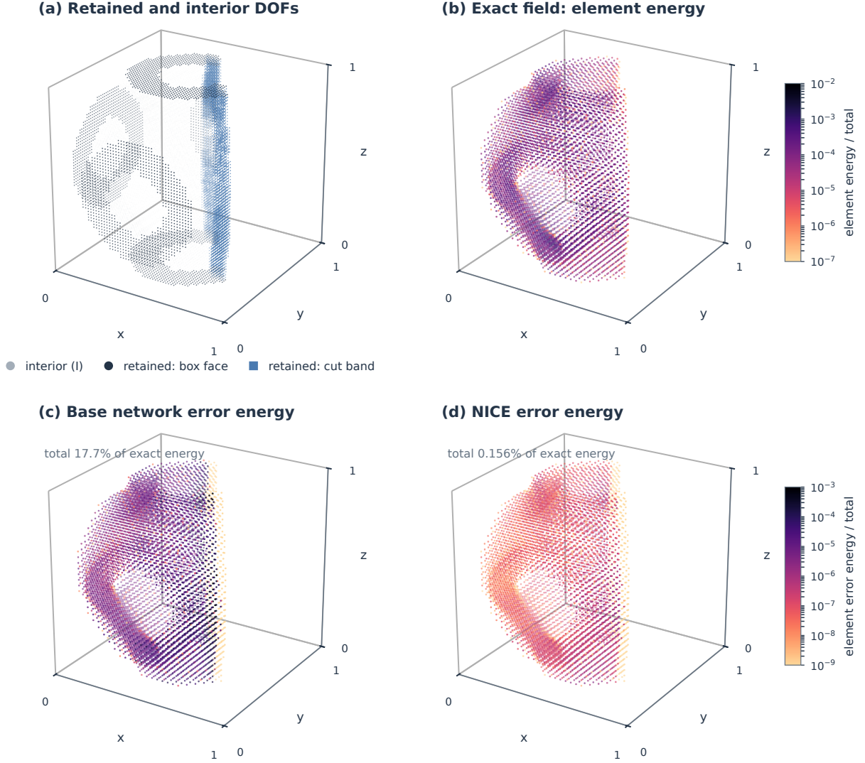
图 7: M1 中的保留自由度及延拓误差的空间分布。(a) 保留胞元界面自由度、保留切割带自由度与内部自由度。(b) 一个一致面力方向下精确场的体单元能量, 相对于其总能量。(c,d) 对相同保留位移, 基础网络与 NICE 误差的体单元能量, 相对于 (b) 中精确场的总能量, 采用统一色标。切割带单元不含误差, 因为其自由度是保留的。
