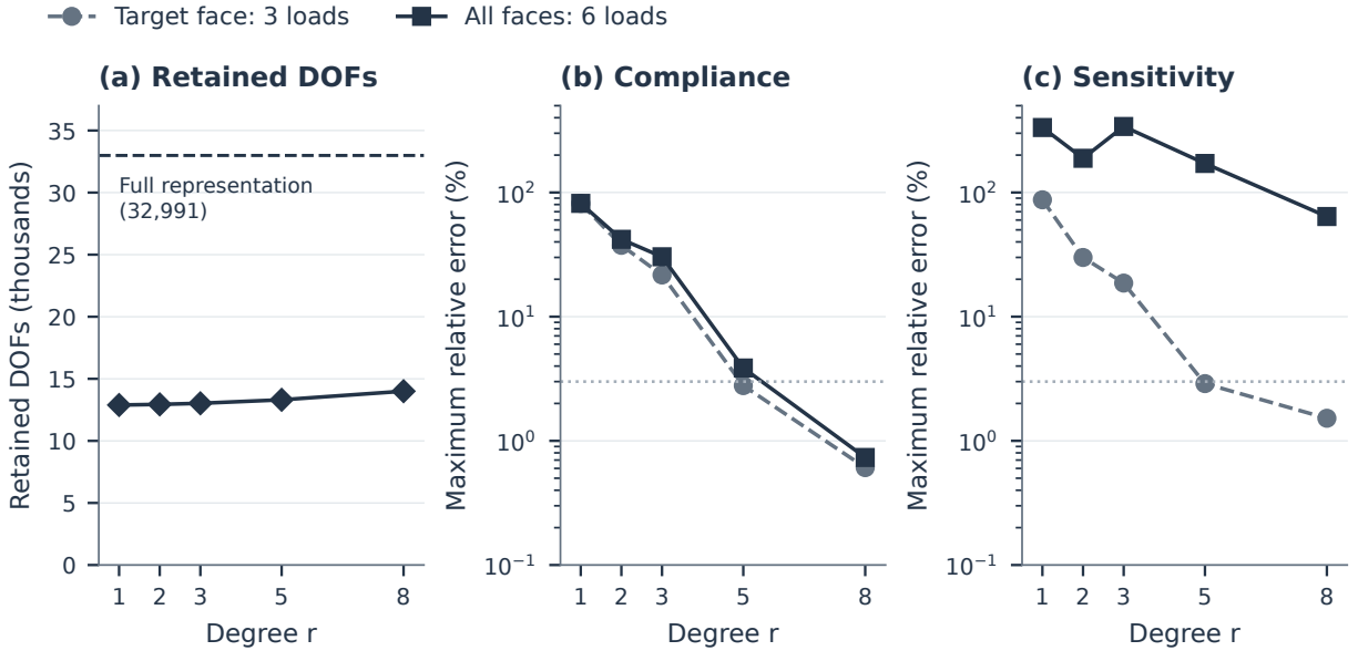
图 12: 限制胞元边界面位移引起的响应误差。H1/x 的两个胞元均采用精确算子，并在每个胞元边界面上采用 r 次 Bernstein 多项式，非胞元边界面切割带自由度不受限制。(a) 保留自由度数目；虚线表示完整表示的 32,991 个自由度。(b,c) 在三个目标面载荷或全部六个目标面与邻胞元面载荷下的最大柔度误差和最大目标胞元灵敏度误差；不计切割面面力。误差相对于完整保留空间解计算；水平线标示 3%。
