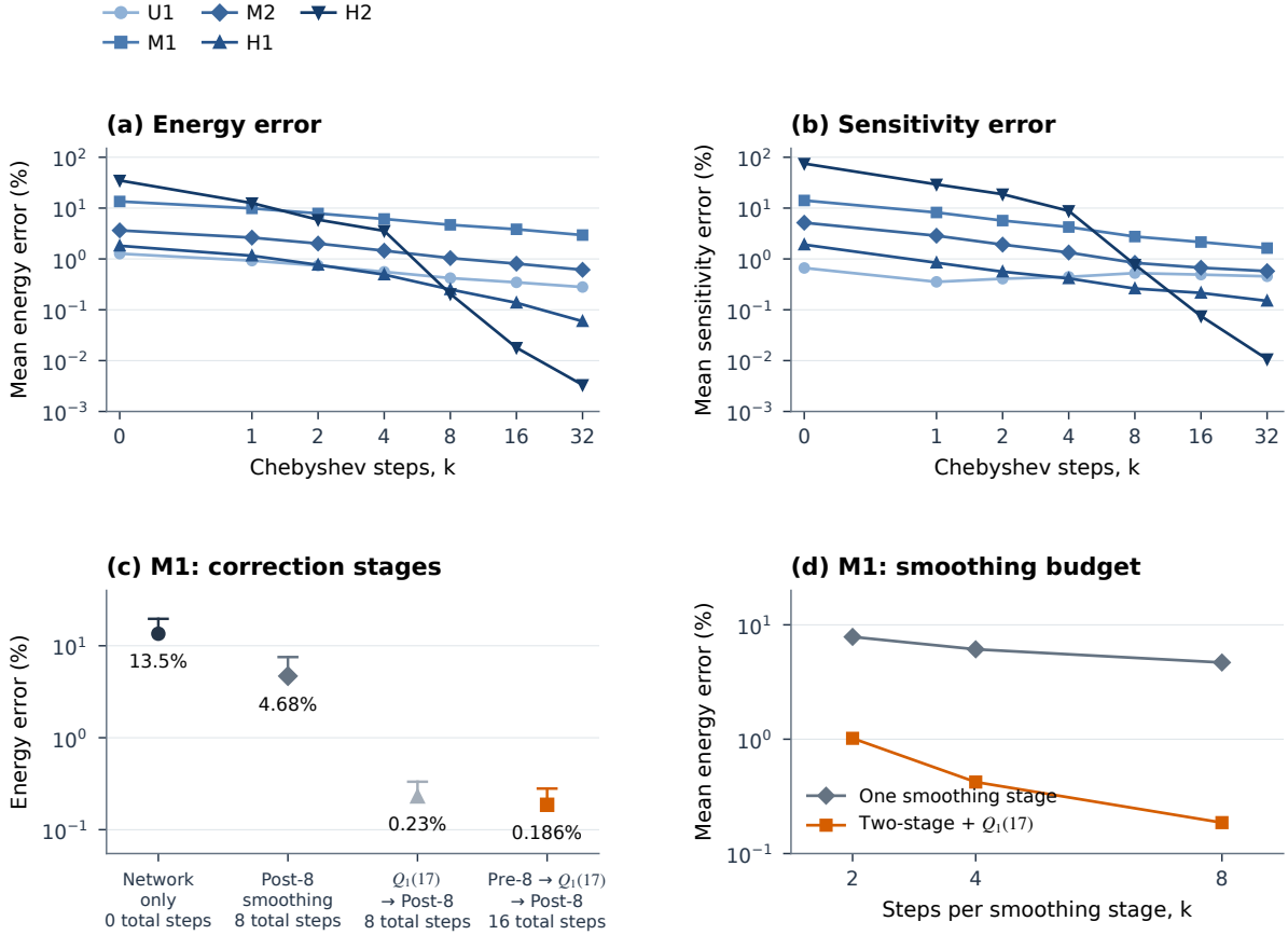
图 8: 在固定网络参数下校正基础网络所获得的精度提升。(a,b) 五个胞元上 Chebyshev 光滑过程中的平均方向能量误差与场基灵敏度误差。(c) M1 在以下情形下的结果: 无校正、八步光滑、粗网格校正后接八步光滑, 以及粗网格校正前后各八步光滑; 圆点表示平均值, 端帽表示第 90 百分位数。(d) M1: 平均能量误差随每个光滑阶段步数 k 的变化, 分别对应单独一个光滑阶段, 以及 k 步前光滑、 Q_1(17) 粗网格校正与 k 步后光滑的组合。所有子图均采用一致面力、固定保留位移以及 a = b/30 ; 在 (a,b) 中, 步数轴在 0 到 1 之间为线性刻度, 此后为对数刻度。
