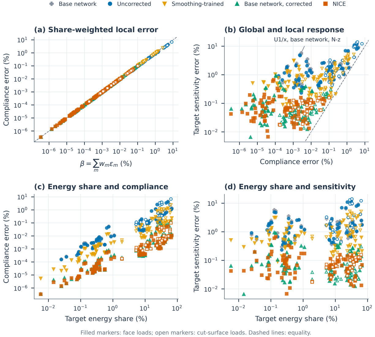
图 11: 按份额加权的柔度误差与局部灵敏度。每个点对应某一变体 - 配置组合的一个载荷；各载荷上的最大值见表 ST08 (面载荷) 和表 ST09 (切割面载荷)。实心标记表示面载荷, 空心标记表示切割面载荷。(a) 柔度误差与 \beta = \sum_m w_m \varepsilon_m 的关系, 其中能量份额 w_m = q_m^T S_m q_m / C , 能量误差 \varepsilon_m = q_m^T (\hat{S}_m - S_m) q_m / (q_m^T S_m q_m) , 均在精确装配保留位移处计算; 只有学习的目标胞元对 \beta 有贡献。(b) 相同载荷下的柔度误差与目标胞元灵敏度误差; 标注指出 U1/x 上邻胞元 z 向载荷下的基础网络。虚线表示相等。(c,d) 两项响应误差随目标胞元精确能量份额的变化。变体同表 2 和图 10。
