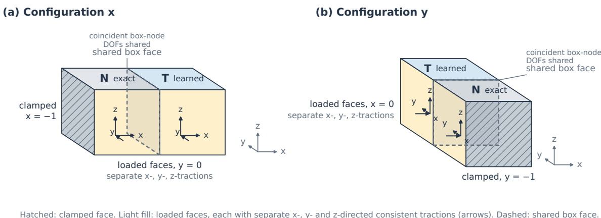
图 9: 两胞元装配的支撑与加载。(a) 配置 x: 邻胞元平移 (-1, 0, 0) ，面 x = -1 固支，面力作用于 y = 0 。(b) 配置 y: 平移为 (0, -1, 0) ，面 y = -1 固支，面力作用于 x = 0 。目标胞元 (T) 面与邻胞元 (N) 面各自分别承受 x、y、z 方向的一致面力载荷。重合的胞元界面节点自由度在界面上共享；非胞元边界面的切割带自由度保持局部。切割目标胞元还承受三个切割面面力，单独分析。
