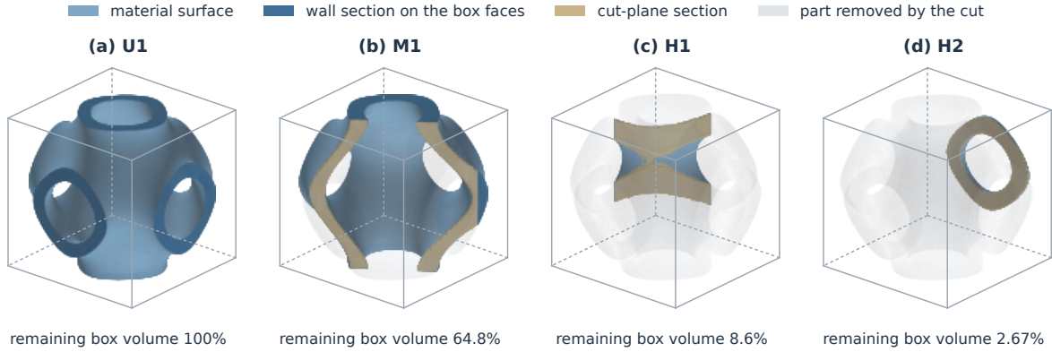
图 4: 代表性验证几何 。(a) 未切割 U1、(b) 中度切割 M1 以及 (c,d) 重度切割 H1 和 H2 采用相同的单位立方体尺度与观察方向。浅蓝色表示材料表面，深蓝色表示胞元边界面上的壁截面，沙色表示切割平面上的截面；被切去的部分以半透明灰色绘出，观察方向朝向切割面一侧。百分比表示切割后剩余的立方体体积相对于单位立方体的比例，未与薄壁材料求交。表面由式 (1) 在每轴 129 个位置的网格上重构，仅用于可视化。
