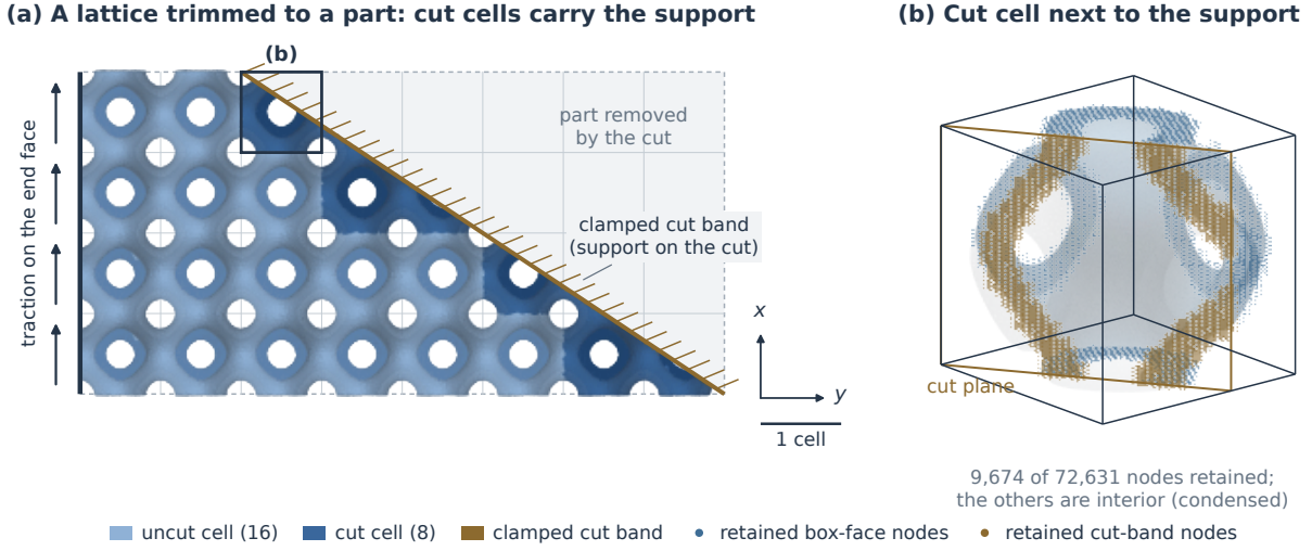
图 1: 修剪为零件形状的点阵，其切割胞元承担支撑。(a) 由 8 \times 4 个 Schwarz-P 胞元（式 (1)，均匀 \tau = 0.40 ）组成的单层被一个平面修剪后的俯视图：16 个未切割胞元（浅色）和 8 个切割胞元（深色）；被切去的部分以浅色虚线框绘出。板经切割处固支：每个切割胞元切割带的全部自由度均被固定（阴影线）。端面承受合力为单位值的面内面力（箭头）。(b) (a) 中框出的切割胞元，壁面半透明并标出切割平面：其 Q_2 模型的 72,631 个节点中，胞元边界面上（蓝色）和切割带中（砂色）的 9,674 个节点被保留，其余均为内部节点，经凝聚消去。曲面由式 (1) 重构，仅用于显示。
