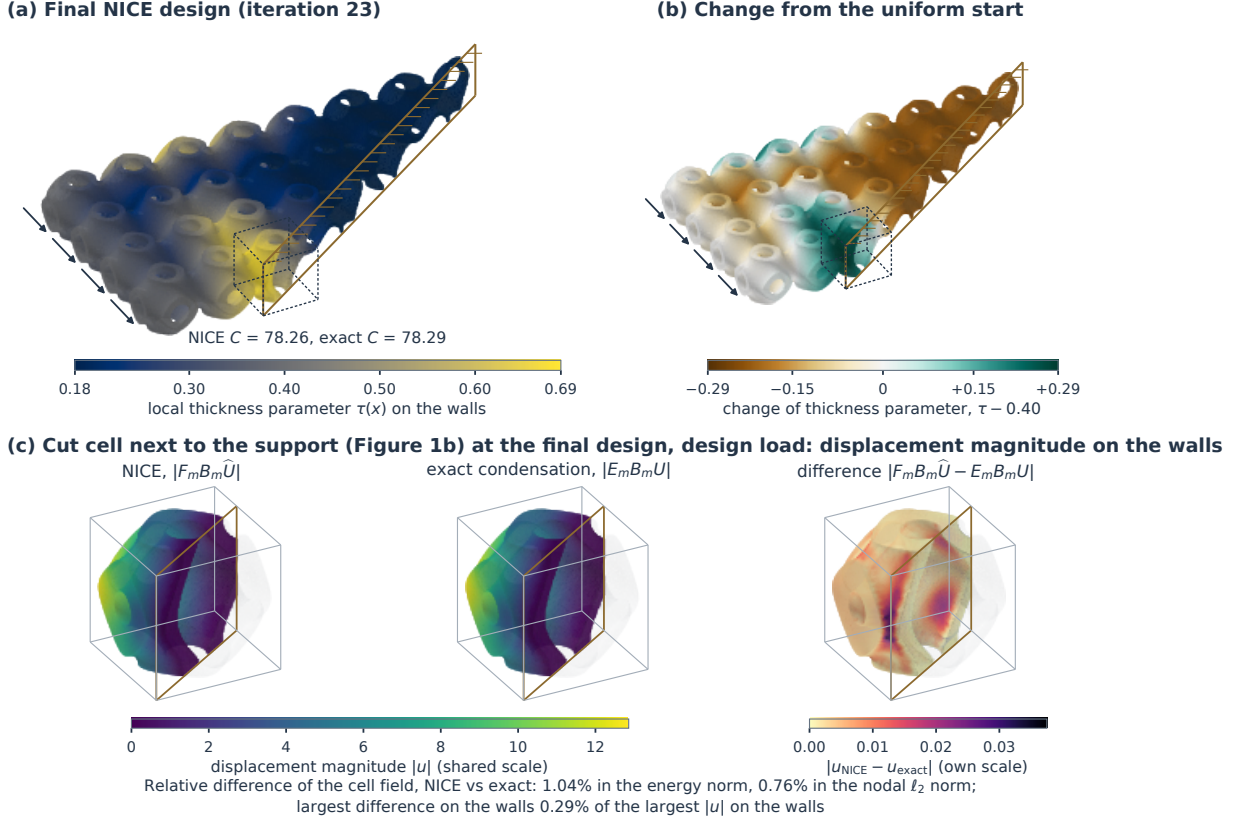
图 13: 经切割带固支的板的厚度设计。(a) NICE 最终设计，壁面按局部厚度参数着色，并标出 NICE 与精确柔度 (表 ST21)。(b) 相对均匀初始设计的变化 \tau - 0.40 ：材料向加载端附近、紧邻支撑的胞元集中 (最多 +0.29)，远离载荷的胞元则被减薄 (最多 -0.22)。(c) 图 1b 中的切割胞元在最终设计和设计载荷下的情况：NICE 恢复场 F_m B_m \hat{U} 与精确凝聚 E_m B_m U 在壁面上的位移大小 (同一色标)，以及二者之差 (单独色标)。两场在该胞元能量范数下相差 1.04%，在节点位移欧氏范数下相差 0.76%；将同一延拓作用于精确保留位移，同样得到 1.04%，因此差异来自局部延拓。在整块板上，能量范数差为 1.72%，其平方等于柔度相对差 2.96 \times 10^{-4} (式 (6))。
