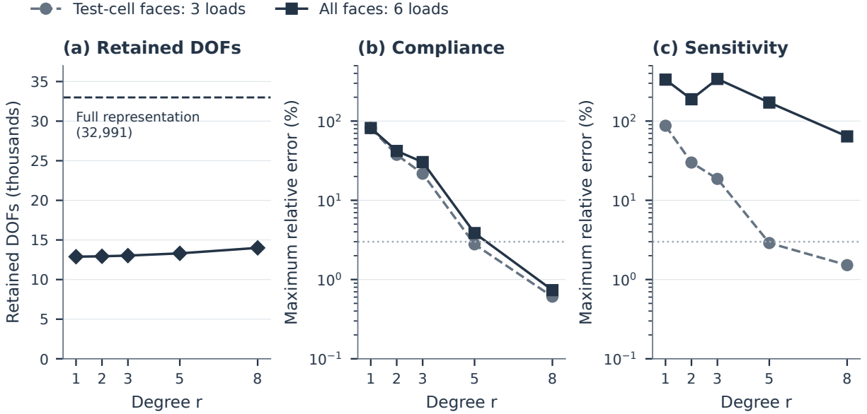
图 12: 限制胞元表面位移引起的响应误差。H1/x 的两个胞元均采用精确凝聚刚度矩阵，并在每个胞元表面上采用 r 次 Bernstein 多项式。切割平面单元中不在胞元表面上的自由度不受限制。(a) 主自由度数目；虚线表示完整表示的 32,991 个自由度。(b,c) 被测胞元表面三个载荷下或被测胞元与相邻胞元表面全部六个载荷下的最大柔度误差和最大被测胞元灵敏度误差。不计切割面上的面力载荷。误差以采用全部主自由度的解为基准，水平线标示 3%。
