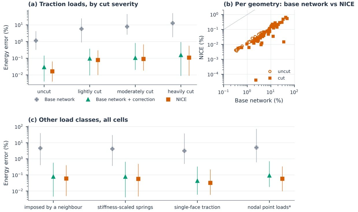
图 5: 基础网络、基础网络加修正与 NICE 在 80 个验证几何上的能量误差。每个观测值为某一几何在某一载荷类别全部验证测试位移上的平均能量误差 q^T(\hat{S} - S)q / (q^T S q) 。(a) 面力载荷，每个切割程度分组 20 个几何。标记表示各几何的均值，误差棒表示第 10 百分位数至最大值的范围。(b) 面力载荷下基础网络与 NICE 的单个几何平均误差。空心标记表示未切割几何，实心标记表示切割几何；点线表示二者相等。(c) 相邻胞元施加的边界位移、按刚度缩放的弹簧支撑、单个表面上的面力载荷以及等值的集中节点载荷。前两类采用 75 个几何，后两类采用 80 个几何。星号标注用作严苛条件检验的集中节点载荷类别。其中二十个几何（6 个未切割，14 个切割）用于检查点选择。变体见表 2；“基础网络加修正”指部署时施加修正而不重新训练的基础网络。
