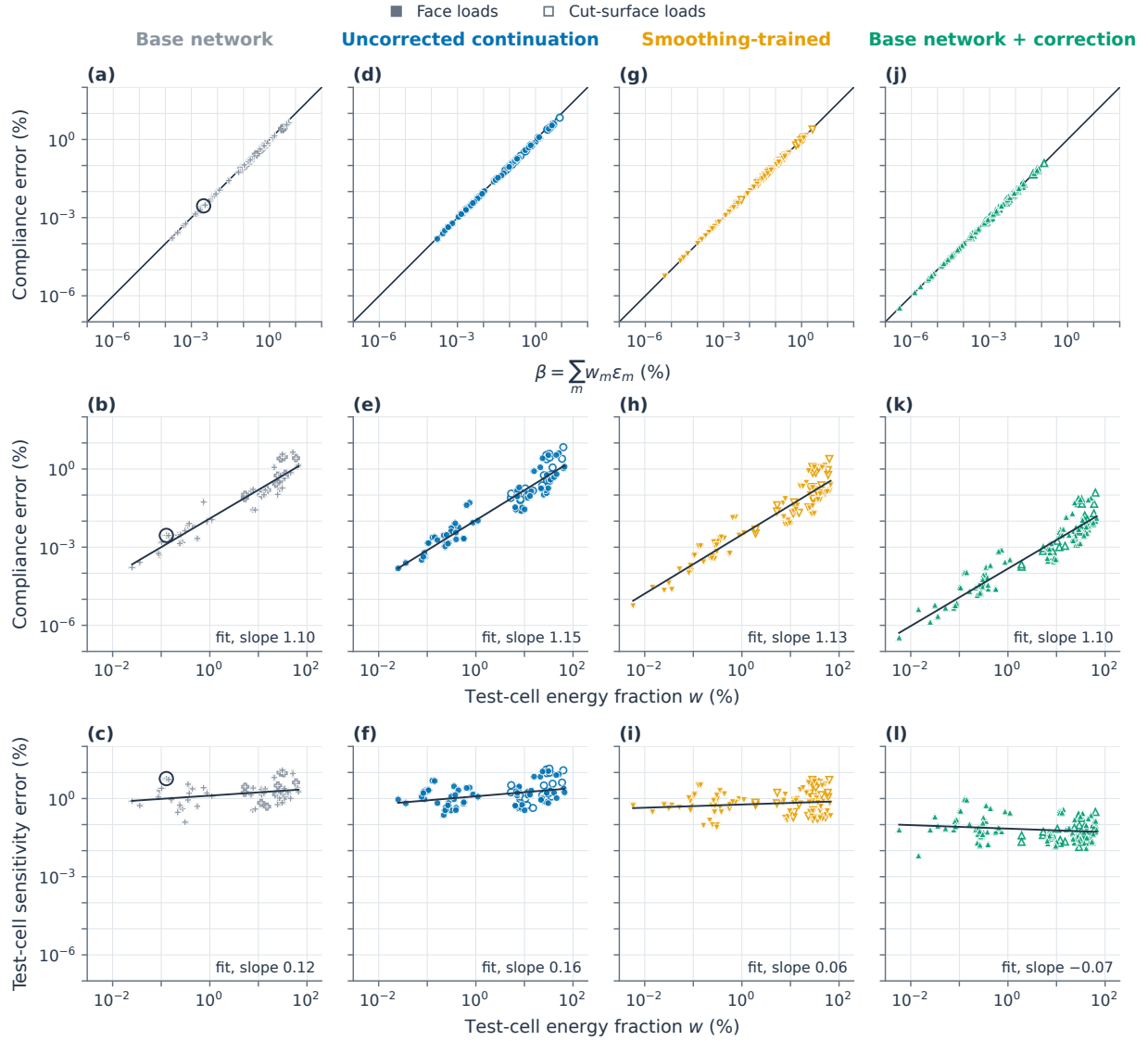
图 S04: 其余四个变体遵循图 11 中的关系。与图 11 相对应, (a–c) 为基础网络, (d–f) 为未修正延续, (g–i) 为平滑训练变体, (j–l) 为基础网络加修正 (部署时施加修正)。每个点对应各变体所评估构型中的一个载荷 (分别为 54、87、96 和 114 个载荷; 表 ST08 和表 ST09); 实心标记表示面载荷, 空心标记表示切割面载荷。第一行: 柔度误差与 \beta 的关系; 直线表示相等。四个变体的柔度误差与 \beta 之比分别介于 0.80–0.98、0.79–0.99、0.92–0.99 和 0.96–1.006 之间; 比值高于 1 的六个载荷, 其超出量至多为柔度的 1.3 \times 10^{-9} 。第二行和第三行: 柔度误差和被测胞元灵敏度误差随被测胞元精确应变能占比 w 的变化; 直线为对数坐标下的最小二乘拟合, 各子图中标出其斜率。所有子图共用误差坐标轴。(a–c) 中圈出的载荷为 U1/x 在相邻胞元表面 z 向面力载荷作用下的情形, 其数值见表 ST08 的说明。
