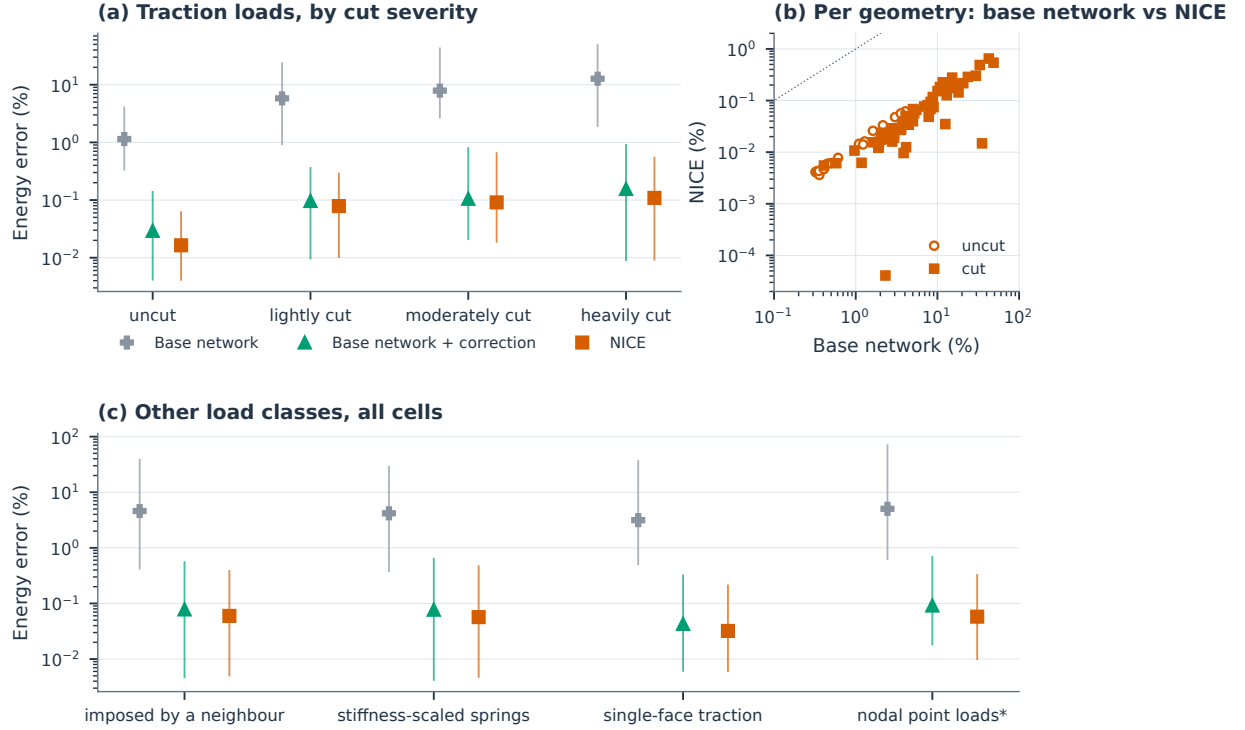
图 5: 基础网络、基础网络加修正与 NICE 在 80 个验证几何上的能量误差。每个观测值为某一几何在某一载荷类别全部验证测试位移上的平均能量误差 q^T(\hat{S} - S)q / (q^T S q) 。(a) 面力载荷, 每个切割程度分组 20 个几何。标记表示各几何的均值, 误差棒表示第 10 百分位数至最大值的范围。(b) 面力载荷下基础网络与 NICE 的单个几何平均误差。空心标记表示未切割几何, 实心标记表示切割几何; 点线表示二者相等。(c) 相邻胞元施加的边界位移、按刚度缩放的弹簧支撑、单个表面上的面力载荷以及等值的集中节点载荷。前两类采用 75 个几何, 后两类采用 80 个几何。星号标注用作严苛条件检验的集中节点载荷类别。其中二十个几何 (6 个未切割, 14 个切割) 用于检查点选择。变体见表 2; “基础网络加修正”指部署时施加修正而不重新训练的基础网络。
