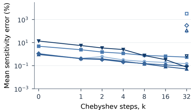
(d) Nodal force: sensitivity
