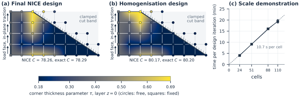
图 15: 板设计与规模演示。(a,b) 最终 NICE 设计与均匀化设计的角点厚度参数, 长边水平绘制, 层 z = 0 ; 圆: 设计变量; 方块: 位于加载面平面内、保持固定的顶点; 绘于移除区域内的顶点为切割胞元的角点。带阴影线的粗线: 固支切割带; 箭头: 加载面及面内面力方向。(c) 在与 (a,b) 中板比例和切割方式相同、沿未切割长边固支并在相对面上施加面内载荷的板上进行的规模演示: 每次设计迭代的时间 (平均值; 误差条: 各计时迭代的范围) 随胞元数的变化; 虚线: 按每胞元平均时间的正比关系; 内存见表 ST20。(a,b) 中的柔度: 同一设计的 NICE 值与精确值 (表 ST21)。
