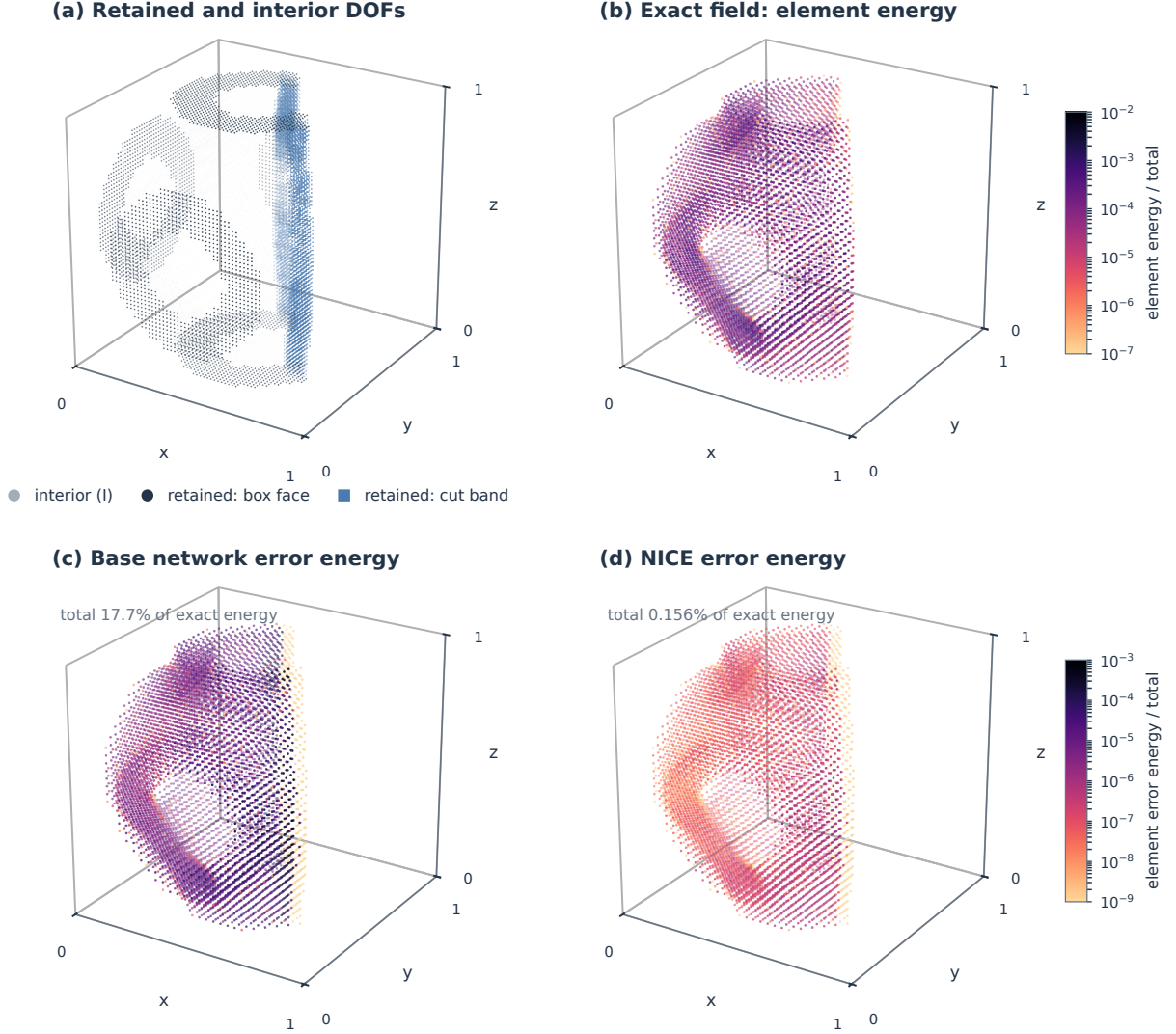
图 7: M1 中的保留自由度及延拓误差的空间分布。(a) 保留胞元边界面自由度、保留切割带自由度与内部自由度。(b) 一个一致面力方向下精确场的体单元能量，相对于其总能量。(c,d) 对相同保留位移，基础网络与 NICE 误差的体单元能量，相对于 (b) 中精确场的总能量，采用统一色标。切割带单元不含误差，因为其自由度是保留的。
