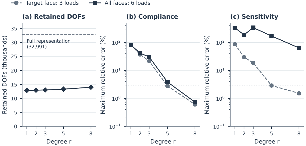
图 12: 限制胞元边界面位移引起的响应误差。H1/x 的两个胞元均采用精确算子, 并在每个胞元边界面上采用 r 次 Bernstein 多项式, 非胞元边界面切割带自由度不受限制。(a) 保留自由度数目; 虚线表示完整表示的 32,991 个自由度。(b,c) 在三个目标面载荷或全部六个目标面与邻胞元面载荷下的最大柔度误差和最大目标胞元灵敏度误差; 不计切割面面力。误差相对于完整保留空间解计算; 水平线标示 3%。
