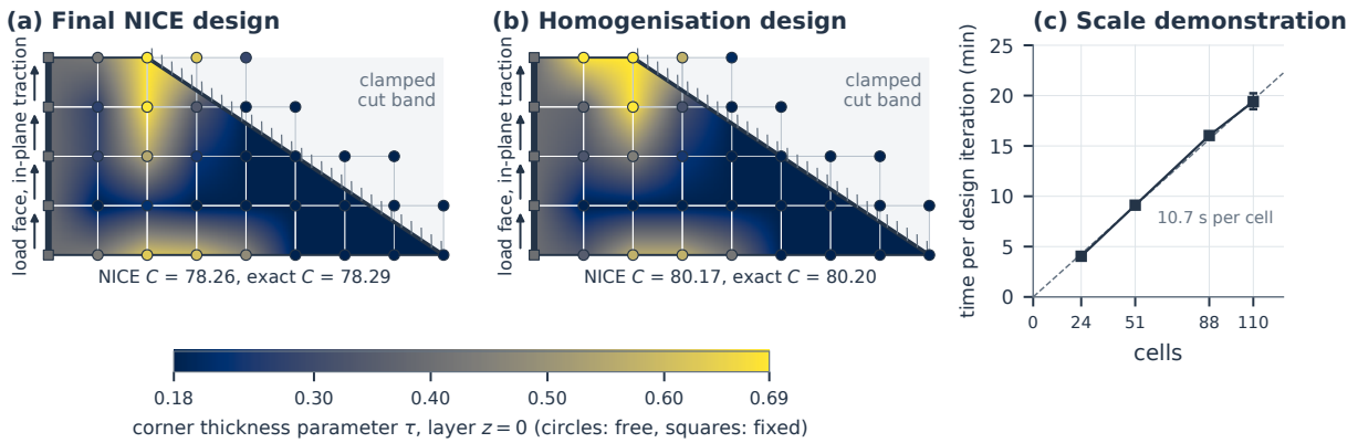
图 15: 板设计与规模演示。(a,b) 最终 NICE 设计与均匀化设计的角点厚度参数, 长边水平绘制, 层 z = 0 ; 圆: 设计变量; 方块: 位于加载面平面内、保持固定的顶点; 绘于移除区域内的顶点为切割胞元的角点。带阴影线的粗线: 固支切割带; 箭头: 加载面及面内面力方向。(c) 在与 (a,b) 中板比例和切割方式相同、沿未切割长边固支并在相对面上施加面内载荷的板上进行的规模演示: 每次设计迭代的时间 (平均值; 误差条: 各计时迭代的范围) 随胞元数的变化; 虚线: 按每胞元平均时间的正比关系; 内存见表 ST20。(a,b) 中的柔度: 同一设计的 NICE 值与精确值 (表 ST21)。
