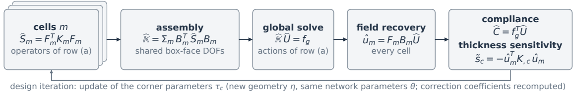
图 2: 学习位移延拓、平衡校正与变分装配。(a) 在由网络延拓变形之前, 先从保留位移中分离出刚体运动。随后重构刚体场并恢复给定的保留值; 校正 \mathcal{W} 接着在固定保留位移下减小内部不平衡, 再施加局部刚度和完整延拓的转置 F^T , 即得到功共轭的保留力。(a) 中的排序即命题 4; 它针对能量误差, 而非灵敏度误差。(b) 各胞元算子在共享胞元边界界面自由度上装配, 并求解装配系统; 装配解为局部场恢复、柔度和场基厚度灵敏度提供输入。一次设计迭代更新角点厚度参数, 从而重新生成每个胞元的几何; 网络参数保持不变, 而 \mathcal{W} 的系数则重新计算。
