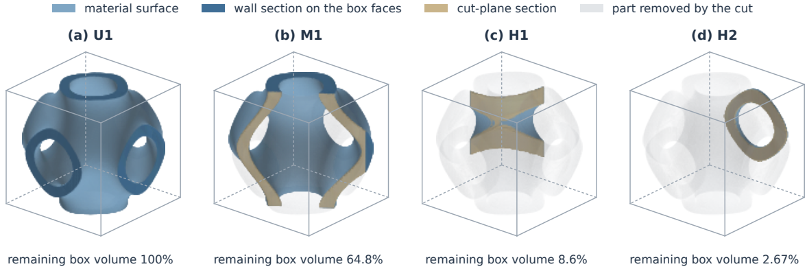
图 4: 代表性验证几何。(a) 未切割 U1、(b) 中度切割 M1 以及 (c,d) 重度切割 H1 和 H2 采用相同的单位立方体尺度与观察方向。浅蓝色表示材料表面, 深蓝色表示胞元边界面上的壁截面, 沙色表示切割平面上的截面; 被切去的部分以半透明灰色绘出, 观察方向朝向切割面一侧。百分比表示切割后剩余的立方体体积相对于单位立方体的比例, 未与薄壁材料求交。表面由式 (1) 在每轴 129 个位置的网格上重构, 仅用于可视化。
