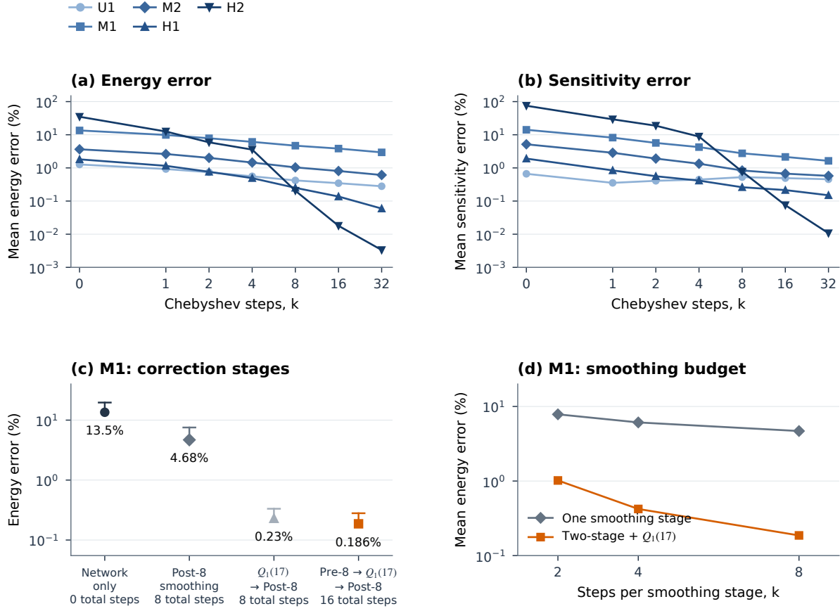
图 8: 在固定网络参数下校正基础网络所获得的精度提升。(a,b) 五个胞元上 Chebyshev 光滑过程中的平均方向能量误差与场基灵敏度误差。(c) M1 在以下情形下的结果：无校正、八步光滑、粗网格校正后接八步光滑，以及粗网格校正前后各八步光滑；圆点表示平均值，端帽表示第 90 百分位数。(d) M1：平均能量误差随每个光滑阶段步数 k 的变化，分别对应单独一个光滑阶段，以及 k 步前光滑、 Q_1(17) 粗网格校正与 k 步后光滑的组合。所有子图均采用一致面力、固定保留位移以及 a = b/30 ；在 (a,b) 中，步数轴在 0 到 1 之间为线性刻度，此后为对数刻度。
