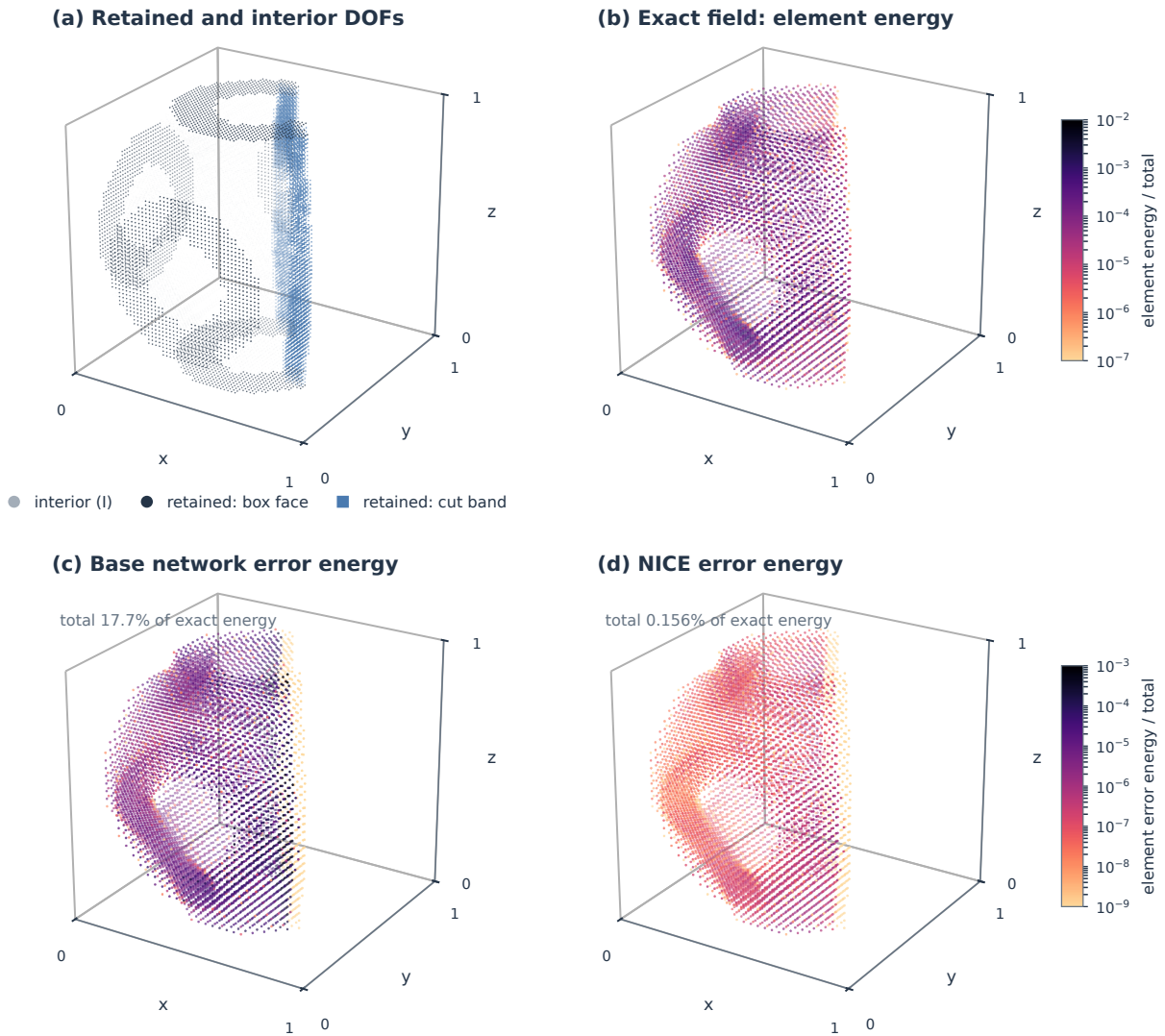
图 7: M1 中的保留自由度及延拓误差的空间分布。(a) 保留胞元边界面自由度、保留切割带自由度与内部自由度。(b) 一个一致面力方向下精确场的体单元能量, 相对于其总能量。(c,d) 对相同保留位移, 基础网络与 NICE 误差的体单元能量, 相对于 (b) 中精确场的总能量, 采用统一色标。切割带单元不含误差, 因为其自由度是保留的。
