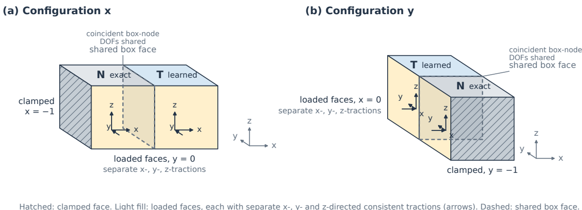
图 9: 两胞元装配的支撑与加载。(a) 配置 x: 邻胞元平移 (-1, 0, 0) ，面 x = -1 固支，面力作用于 y = 0 。(b) 配置 y: 平移为 (0, -1, 0) ，面 y = -1 固支，面力作用于 x = 0 。目标胞元 (T) 面与邻胞元 (N) 面各自分别承受 x、y、z 方向的一致面力载荷。重合的胞元边界面节点自由度在界面上共享；非胞元边界面的切割带自由度保持局部。切割目标胞元还承受三个切割面面力，单独分析。
