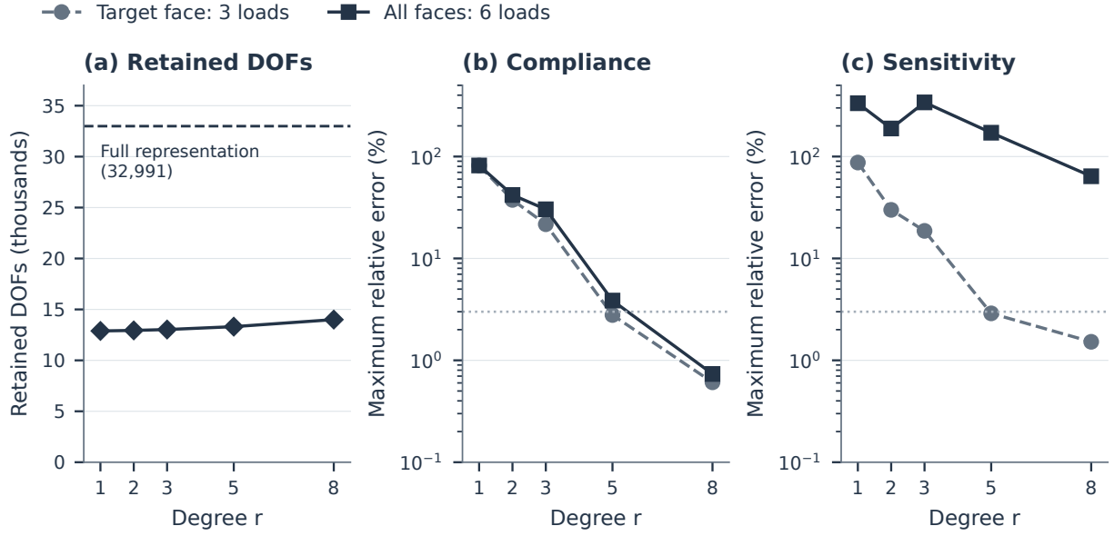
图 12: 限制胞元边界面位移引起的响应误差。H1/x 的两个胞元均采用精确算子, 并在每个胞元边界面上采用 r 次 Bernstein 多项式, 非胞元边界面切割带自由度不受限制。(a) 保留自由度数; 虚线表示完整表示的 32,991 个自由度。(b,c) 在三个目标面载荷或全部六个目标面与邻胞元面载荷下的最大柔度误差和最大目标胞元灵敏度误差; 不计切割面面力。误差相对于完整保留空间解计算; 水平线标示 3%。
