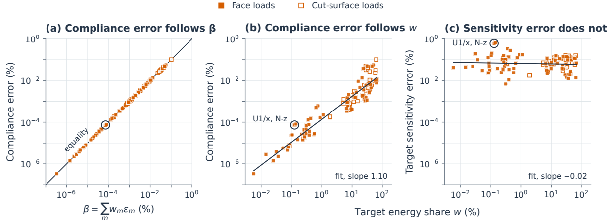
图 11: 柔度误差按能量份额折减, 灵敏度误差不折减。NICE 在七个选择胞元的十四种配置中的结果, 每个点对应一个载荷: 84 个面载荷 (实心标记) 和 30 个切割面载荷 (空心标记); 各载荷上的最大值见表 ST08 和表 ST09。(a) 柔度误差与 \beta = \sum_m w_m \varepsilon_m 的关系, 其中能量份额 w_m = q_m^T S_m q_m / C , 能量误差 \varepsilon_m = q_m^T (\hat{S}_m - S_m) q_m / (q_m^T S_m q_m) , 均在精确装配保留位移处计算; 只有学习的目标胞元对 \beta 有贡献。直线表示相等。对每个载荷, 柔度误差均为 \beta 的 0.963 至 1.004 倍; 比值高于 1 的五个载荷, 其超出量至多为柔度的 7.8 \times 10^{-10} , 而胞元对求解的残差功可达柔度的 1.8 \times 10^{-8} (补充说明 S4.3)。(b) 柔度误差和 (c) 目标胞元灵敏度误差随目标胞元精确能量份额 w 的变化; 实线为对数坐标下的最小二乘拟合。圈出的载荷为 U1/x 上的邻胞元面 z 向面力 (表 5)。其余四个变体见图 S04。
