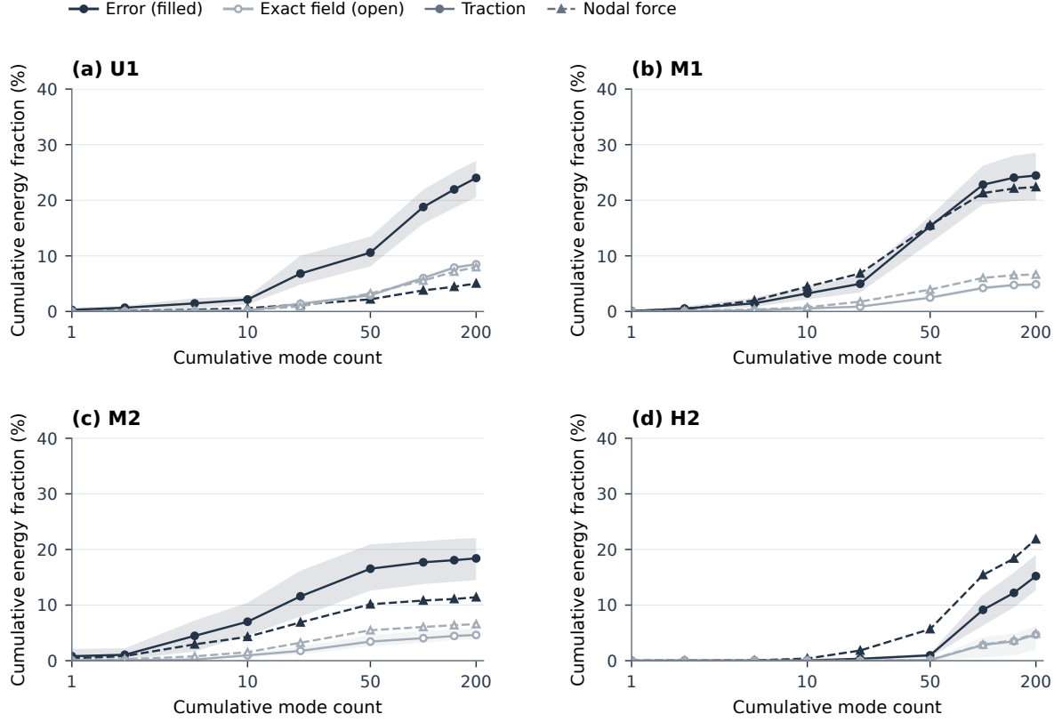
图 6: 基础网络延拓误差的谱分布。各子图分别给出基础网络在 U1、M1、M2 和 H2 上的结果。模态求解 Av = \lambda Dv , 其中 D = \text{diag}(A) , 并按特征值递增排序。深色实心标记表示延拓误差, 浅灰色空心标记表示精确内部场; 实线圆形对应一致面力, 虚线三角形对应节点力。曲线为方向平均值; 色带给出一致面力下第 10–90 方向百分位数。每条累积分数曲线均采用其自身场或误差的内部总能量。
