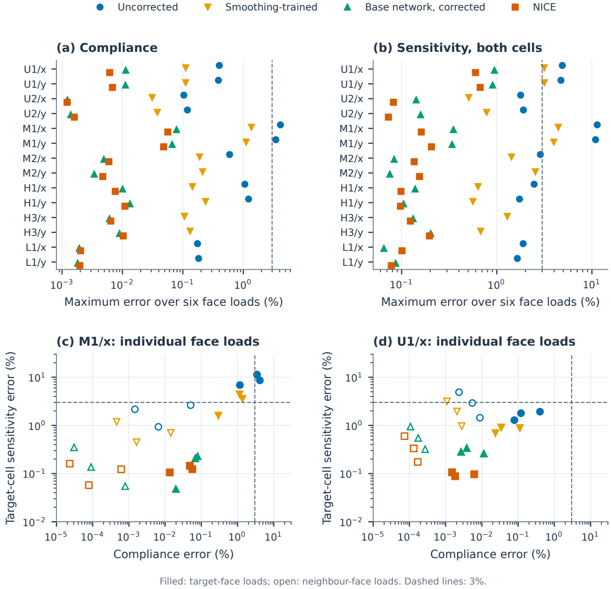
图 10: 两胞元装配中的刚度与厚度灵敏度。目标胞元由学习子结构表示, 邻胞元由精确凝聚表示。(a,b) 每种配置中六个面载荷上的最大误差; 灵敏度误差还在两个胞元上取最大。(c,d) M1/x 与 U1/x 上各单个面载荷的刚度误差与目标胞元灵敏度误差; 实心标记表示目标胞元面载荷, 空心标记表示邻胞元面载荷。虚线标出 3% 线。图中未显示基础网络, 且并非每个变体都在每种配置上进行了评估; 全部结果见表 ST08。变体同表 2; “基础网络 (加校正)” 指在部署时施加校正、未经重新训练的基础网络。
