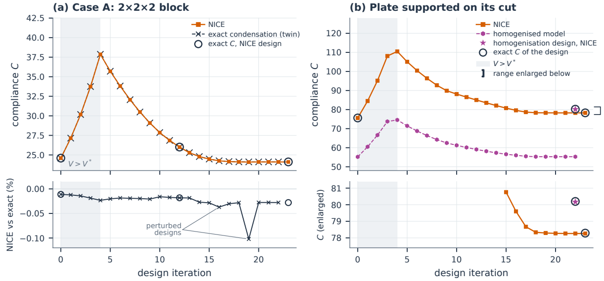
图 14: 基于 NICE 的厚度优化。(a) 算例 A: NICE 优化与采用精确凝聚的孪生优化的柔度历程, 以及 NICE 设计在第 0、12 和 23 次迭代时的精确柔度 (空心圆); 在体积由 1.25V^* 减小至 V^* 的过程中 (阴影, 第 0-3 次迭代), 柔度先上升。下方条带: NICE 柔度相对于同一设计迭代处孪生运行的偏差 (线; 两次运行的设计在第 0-4 次迭代时重合, 此后不同), 以及相对于同一设计精确柔度的偏差 (圆: -0.011\% 、 -0.018\% 、 -0.028\% ); 在第 16 和 19 次迭代 (标注为 'perturbed designs'), 几何生成的回退机制对 NICE 设计施加了扰动 (补充说明 S6.4, 表 ST19a)。(b) 切割面固支板: 从均匀初始设计出发的 NICE 柔度、均匀化宏观模型沿其自身优化路径的柔度 (虚线)、在切割几何上用 NICE 分析的均匀化设计 (星号, 位于最后一次宏观迭代处), 以及均匀初始设计、最终 NICE 设计和均匀化设计的精确柔度 (空心圆)。阴影: V > V^* 的设计迭代。下方条带: 括号所标范围的放大, 自第 15 次迭代起。
