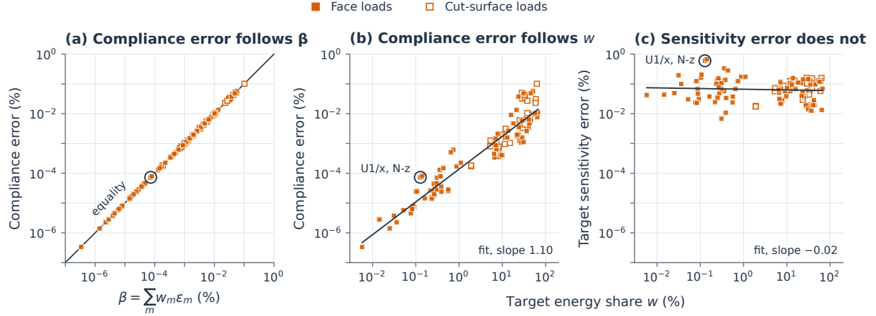
图 11: 柔度误差按能量份额折减, 灵敏度误差不折减。NICE 在七个选择胞元的十四种配置中的结果, 每个点对应一个载荷: 84 个面载荷 (实心标记) 和 30 个切割面载荷 (空心标记); 各载荷上的最大值见表 ST08 和表 ST09。(a) 柔度误差与 \beta = \sum_m w_m \epsilon_m 的关系, 其中能量份额 w_m = q_m^T S_m q_m / C , 能量误差 \epsilon_m = q_m^T (\hat{S}_m - S_m) q_m / (q_m^T S_m q_m) , 均在精确装配保留位移处计算; 只有学习的目标胞元对 \beta 有贡献。直线表示相等。对每个载荷, 柔度误差均为 \beta 的 0.963 至 1.004 倍; 比值高于 1 的五个载荷, 其超出量至多为柔度的 7.8 \times 10^{-10} , 而胞元对求解的残差功可达柔度的 1.8 \times 10^{-8} (补充说明 S4.3)。(b) 柔度误差和 (c) 目标胞元灵敏度误差随目标胞元精确能量份额 w 的变化; 实线为对数坐标下的最小二乘拟合。圈出的载荷为 U1/x 上的邻胞元面 z 向面力 (表 5)。其余四个变体见图 S04。
