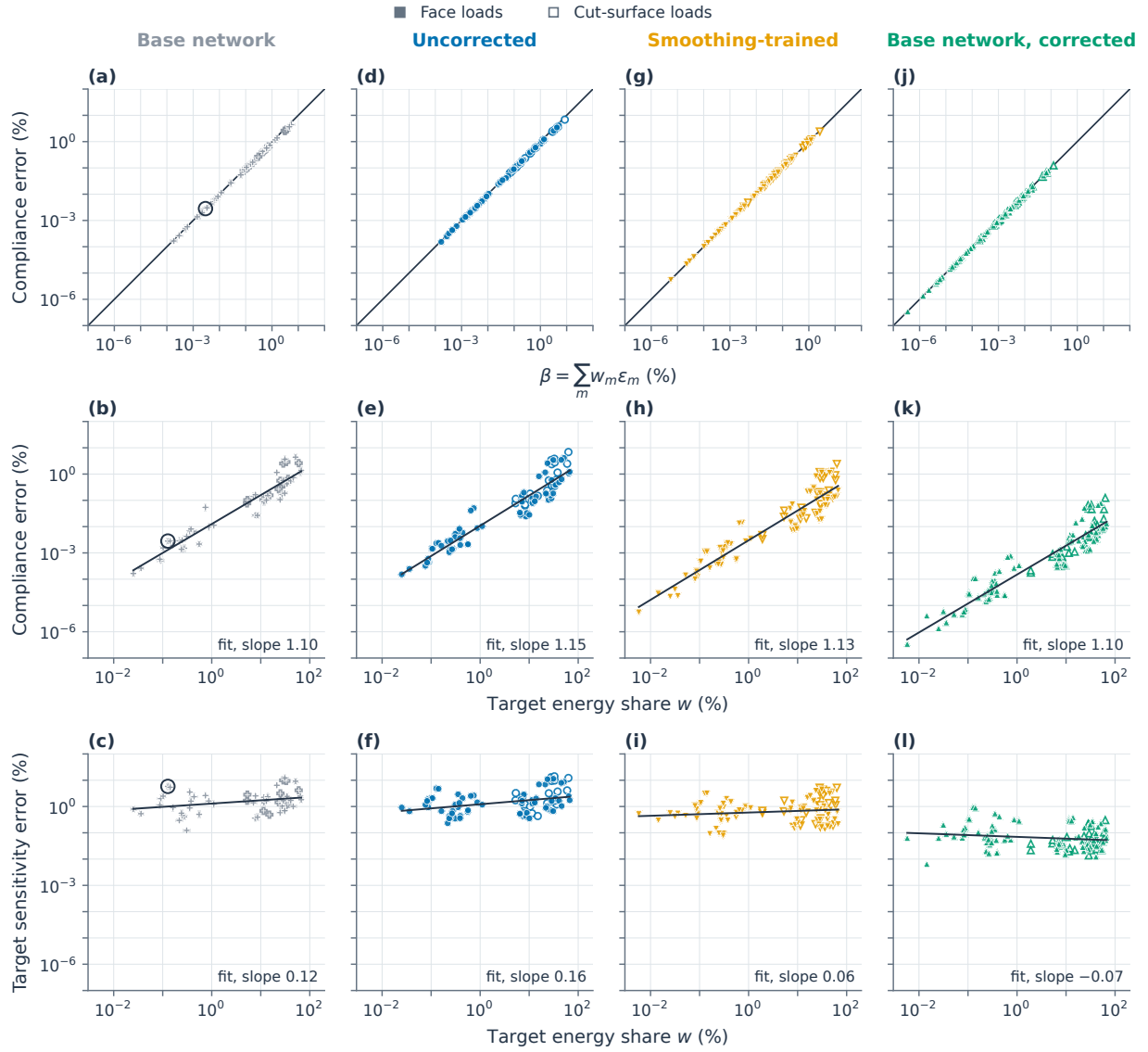
图 S04: 其余四个变体遵循图 11 中的关系。与图 11 相对应, (a-c) 为基础网络, (d-f) 为未校正, (g-i) 为平滑训练, (j-l) 为部署时施加校正的基础网络。每个点对应各变体所评估配置中的一个载荷 (分别为 54、87、96 和 114 个载荷; 表 ST08 和表 ST09); 实心标记表示面载荷, 空心标记表示切割面载荷。第一行: 柔度误差与 \beta 的关系; 直线表示相等。四个变体的柔度误差与 \beta 之比分别介于 0.80–0.98、0.79–0.99、0.92–0.99 和 0.96–1.006 之间; 比值高于 1 的六个载荷, 其超出量至多为柔度的 1.3 \times 10^{-9} 。第二行和第三行: 柔度误差和目标胞元灵敏度误差随目标胞元精确能量份额 w 的变化; 直线为对数坐标下的最小二乘拟合, 各子图中标出其斜率。所有子图共用误差坐标轴。(a-c) 中圈出的载荷为 U1/x 上的邻胞元面 z 向面力, 其数值见表 ST08 的说明。
