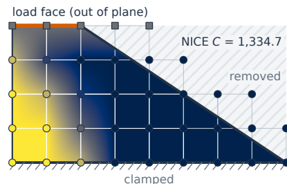
(d) Final design XH_z
