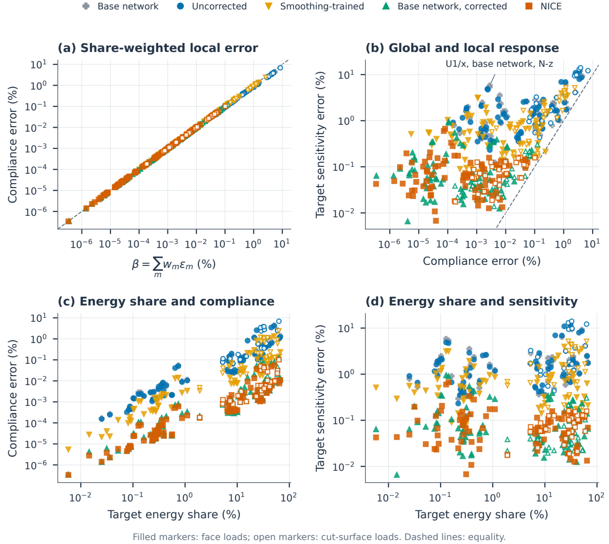
图 10: 按份额加权的柔度误差与局部灵敏度。每个点对应某一变体 - 配置组合的一个载荷；各载荷上的最大值见表 ST08 (面载荷) 和表 ST09 (切割面载荷)。实心标记表示面载荷, 空心标记表示切割面载荷。(a) 柔度误差与 \beta = \sum_m w_m \varepsilon_m 的关系, 其中能量份额 w_m = q_m^T S_m q_m / C , 能量误差 \varepsilon_m = q_m^T (\hat{S}_m - S_m) q_m / (q_m^T S_m q_m) , 均在精确装配保留位移处计算; 只有学习的目标胞对 \beta 有贡献。(b) 相同载荷下的柔度误差与目标胞灵敏度误差; 标注指出 U1/x 上邻胞 z 向载荷下的基础网络。虚线表示相等。(c,d) 两项响应误差随目标胞精确能量份额的变化。变体同表 2 和图 9。
