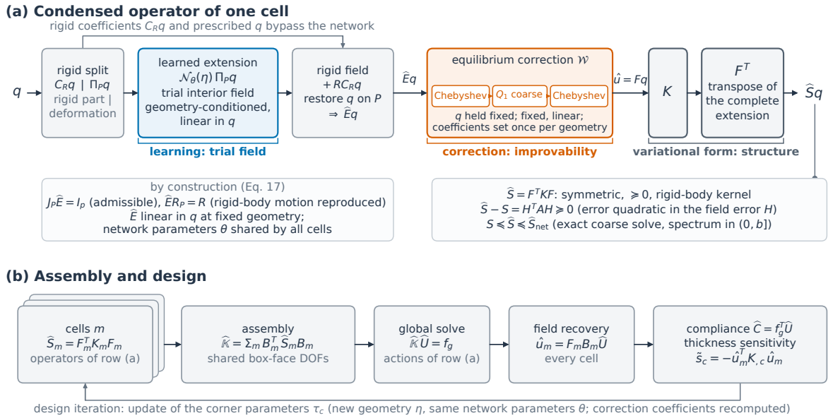
图 2: 学习位移延拓、平衡校正与变分装配。(a) 在由网络延拓变形之前, 先从保留位移中分离出刚体运动。随后重构刚体场并恢复给定的保留值; 校正 \mathcal{W} 接着在固定保留位移下减小内部不平衡, 再施加局部刚度和完整延拓的转置 F^T , 即得到功共轭的保留力。(a) 中的排序假设粗网格校正精确, 且光滑区间的上端界住谱; 它对能量误差排序, 而非对灵敏度误差排序。(b) 各胞算子在共享盒面自由度上装配, 并求解装配系统; 装配解为局部场恢复、柔度和场基厚度灵敏度提供输入。一次设计迭代更新角点厚度参数, 从而重新生成每个胞的几何; 网络参数保持不变, 而 \mathcal{W} 的系数则重新计算。
