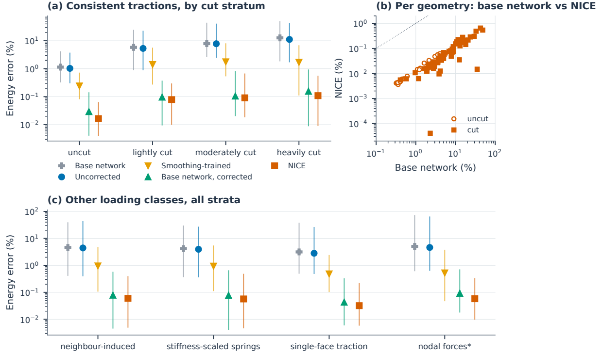
图 4: 学习子结构在 80 个验证几何上的方向能量误差。每个观测值为某一几何在某一载荷类别各验证方向上的平均方向能量误差 q^T(\hat{S} - S)q / (q^T S q) 。(a) 一致面力, 每个切割分层 20 个几何: 标记表示各几何的平均值, 误差棒表示从第 10 百分位数到最大值的范围。(b) 一致面力下基础网络与 NICE 的几何平均值, 空心标记表示未切割几何, 实心标记表示切割几何; 点线表示相等。(c) 邻胞诱导保留位移、刚度缩放弹簧支撑、单面一致面力与等值节点力 (前两类为 75 个几何, 其余为 80 个); 星号标注节点力压力测试。其中二十个几何 (6 个未切割, 14 个切割) 用于检查点选择。变体同表 2; “基础网络 (加校正)” 指在部署时施加校正的基础网络。
