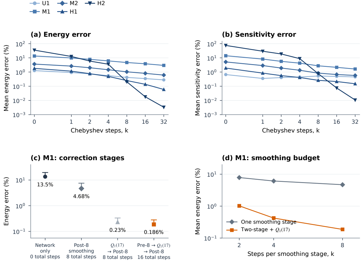
图 7: 在固定网络参数下校正基础网络所获得的精度提升。(a,b) 五个胞上 Chebyshev 光滑过程中的平均方向能量误差与场基灵敏度误差。(c) M1 在以下情形下的结果: 无校正、八步光滑、粗网格校正后接八步光滑, 以及粗网格校正前后各八步光滑; 圆点表示平均值, 端帽表示第 90 百分位数。(d) M1: 平均能量误差随每个光滑阶段步数 k 的变化, 分别对应单独一个光滑阶段, 以及 k 步前光滑、 Q_1(17) 粗网格校正与 k 步后光滑的组合。所有子图均采用一致面力、固定保留位移以及 a = b/30 ; 在 (a,b) 中, 步数轴在 0 到 1 之间为线性刻度, 此后为对数刻度。
