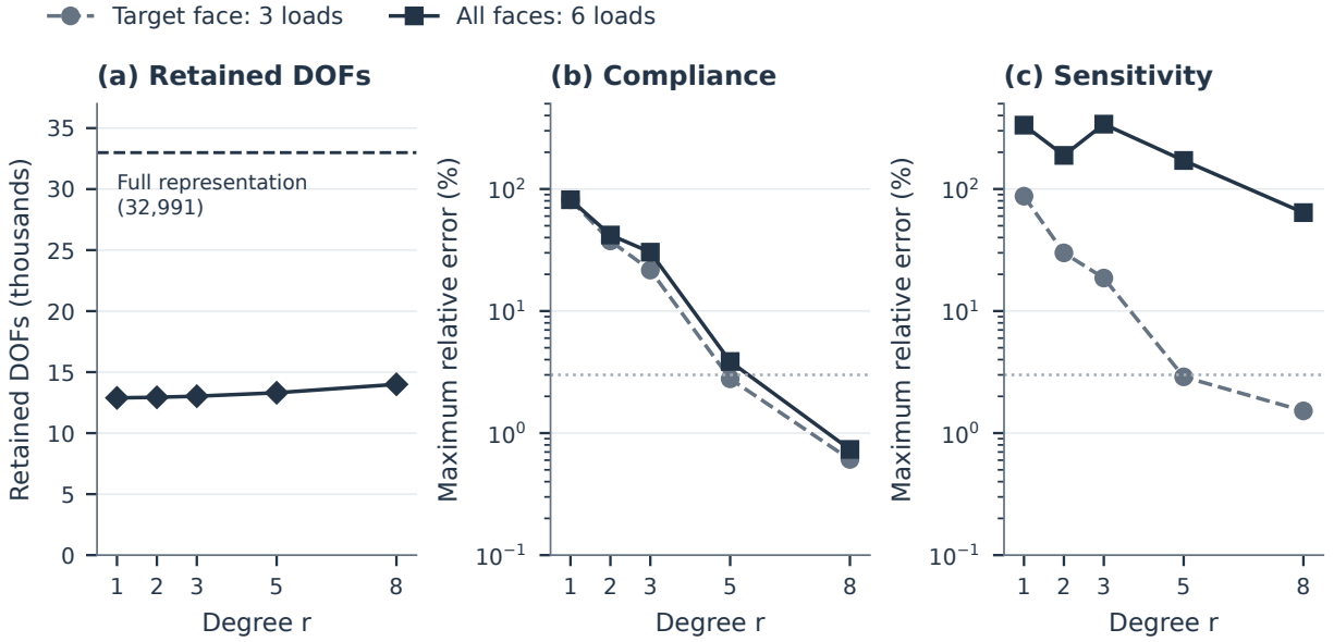
图 11: 限制盒面位移引起的响应误差。H1/x 的两个胞均采用精确算子，并在每个盒面上采用 r 次 Bernstein 多项式，非盒面切割带自由度不受限制。(a) 保留自由度数目；虚线表示完整表示的 32,991 个自由度。(b,c) 在三个目标面载荷或全部六个目标面与邻胞面载荷下的最大柔度误差和最大目标胞灵敏度误差；不计切割面力。误差相对于完整保留空间解计算；水平线标示 3%。
