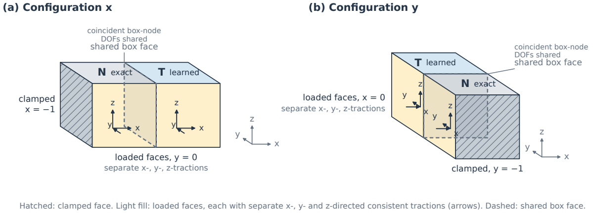
图 8: 两胞装配的支撑与加载。(a) 配置 x : 邻胞平移 (-1, 0, 0) ，面 x = -1 固支，面力作用于 y = 0 。(b) 配置 y : 平移为 (0, -1, 0) ，面 y = -1 固支，面力作用于 x = 0 。目标胞 (T) 面与邻胞 (N) 面各自分别承受 x 、 y 、 z 方向的一致面力载荷。重合的盒节点自由度在界面上共享；非盒面的切割带自由度保持局部。切割目标胞还承受三个切割面面力，单独分析。
