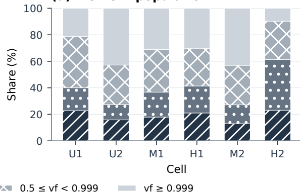
(d) Element population
