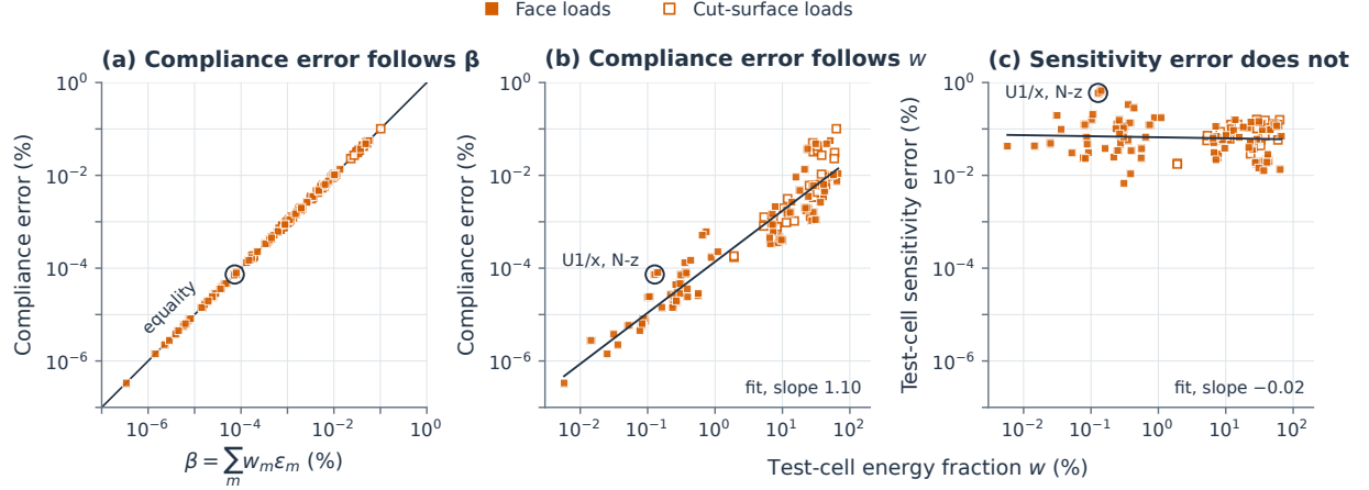
图 11: 柔度误差随被测胞元的应变能占比减小，灵敏度误差则不随之减小。NICE 在七个被测胞元的十四种构型中的结果，每个点对应一个载荷，共有 84 个面载荷（实心标记）和 30 个切割面载荷（空心标记）。各载荷上的最大值见补充表 ST08 和补充表 ST09。(a) 柔度误差与 \beta = \sum_m w_m \varepsilon_m 的关系，其中应变能占比 w_m = q_m^T S_m q_m / C 和能量误差 \varepsilon_m = q_m^T (\hat{S}_m - S_m) q_m / (q_m^T S_m q_m) 均在精确装配的主自由度位移处计算。只有学习的被测胞元对 \beta 有贡献。直线表示二者相等。对每个载荷，柔度误差均为 \beta 的 0.963 至 1.004 倍。比值高于 1 的五个载荷，其超出量至多为柔度的 7.8 \times 10^{-10} ，而胞元对求解的残差功可达柔度的 1.8 \times 10^{-8} （补充说明 S4.3）。(b) 柔度误差和 (c) 被测胞元灵敏度误差随被测胞元精确应变能占比 w 的变化；实线为对数坐标下的最小二乘拟合。圈出的点为 U1/x 在相邻胞元表面 z 向面力载荷下的结果。其余变体的相应结果见图 S04。
