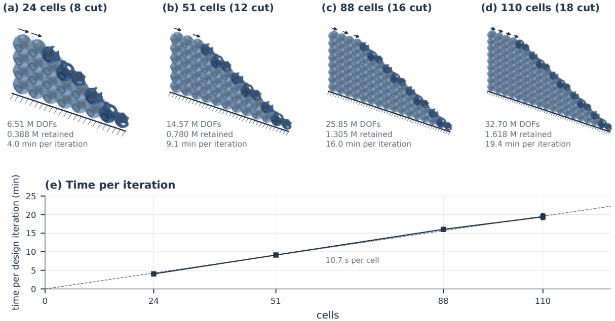
图 16: 规模算例中的板。(a-d) 胞元数为 24、51、88 和 110 的板，长宽比和切割方式与图 15 中的板相同，取均匀初始设计 \tau = 0.40 ，按同一比例绘制。各板立于其固支长边上（阴影线），对面施加沿长边方向的面内面力（箭头）。浅色为未切割胞元，深色为切割胞元。各子图注明切割有限元模型的自由度数、未约束的主自由度数 and 每次设计迭代的平均用时。(e) 每次设计迭代用时随胞元数的变化（方块为平均值，误差棒为所计时迭代的范围）。虚线与胞元数成正比，对应平均每个胞元 10.7 s。内存占用见补充表 ST20。
