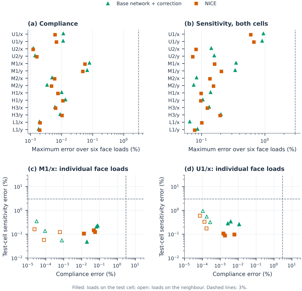
图 10: 两胞元装配中的柔度与厚度灵敏度。被测胞元采用学习子结构表示, 相邻胞元采用精确静力凝聚表示。图中给出 NICE 和基础网络加修正的结果, 后者指部署时施加修正而不重新训练的基础网络。(a,b) 每种构型中六个面载荷上的最大误差; 灵敏度误差还取两个胞元上的最大值。(c,d) M1/x 和 U1/x 上各面载荷下的柔度误差与被测胞元灵敏度误差。实心标记表示施加于被测胞元表面的载荷, 空心标记表示施加于相邻胞元表面的载荷。虚线标示 3%。全部结果见补充表 ST08。该表还包括基础网络和补充说明 S8 中两种变体的结果, 这三者并未在每种构型上都经过评估。
