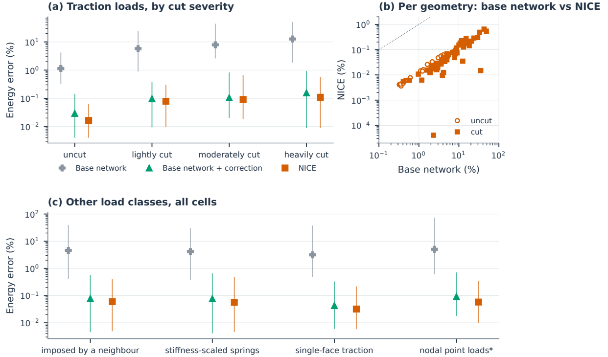
图 5: 基础网络、基础网络加修正与 NICE 在 80 个验证几何上的能量误差。每个观测值为某一几何在某一载荷类别全部验证测试位移上的平均能量误差 q^T(\hat{S} - S)q / (q^T S q) 。(a) 面力载荷，每个切割程度分组 20 个几何。标记表示各几何的均值，误差棒表示第 10 百分位数至最大值的范围。(b) 面力载荷下基础网络与 NICE 的单个几何平均误差。空心标记表示未切割几何，实心标记表示切割几何；点线表示二者相等。(c) 相邻胞元施加的边界位移、按刚度缩放的弹簧支撑、单个表面上的面力载荷以及等值的集中节点载荷。前两类采用 75 个几何，后两类采用 80 个几何。星号标注用作严苛条件检验的集中节点载荷类别。其中二十个几何（6 个未切割，14 个切割）用于检查点选择。变体见表 2；“基础网络加修正”指部署时施加修正而不重新训练的基础网络。
