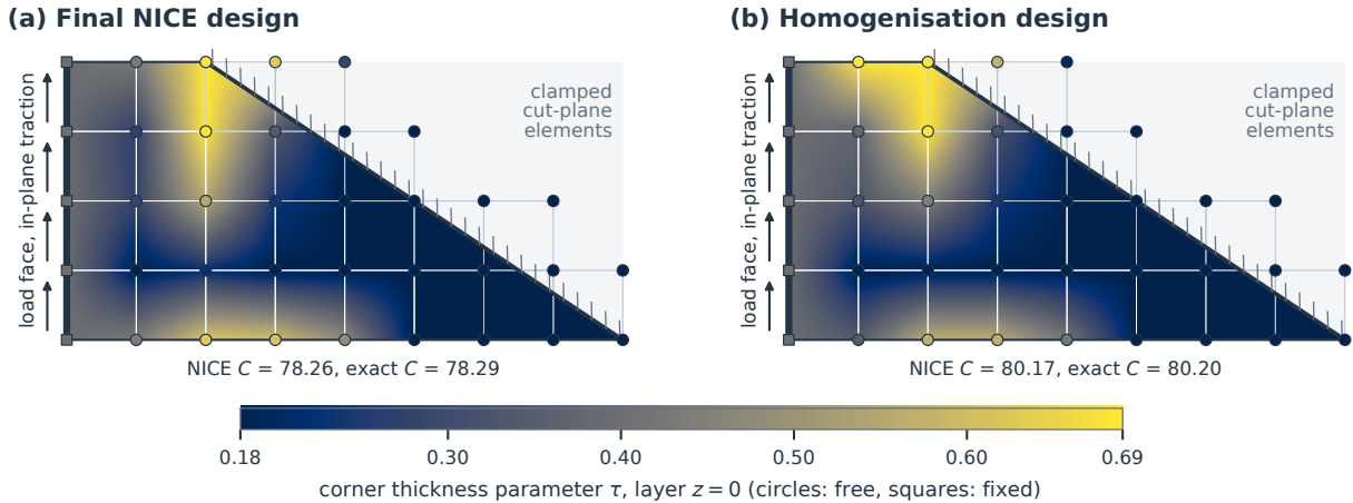
图 15: 切割面固支板的设计。(a,b) 最终 NICE 设计与均匀化设计在层 z = 0 中的角点厚度参数, 长边水平绘制。圆表示设计变量, 方块表示加载面所在平面内保持固定的顶点。绘于切除区域内的顶点为切割胞元的角点。带阴影线的粗线表示固支的切割平面单元, 箭头表示加载面及面内面力的方向。(a,b) 中的柔度为同一设计的 NICE 值与精确值 (补充表 ST21)。
