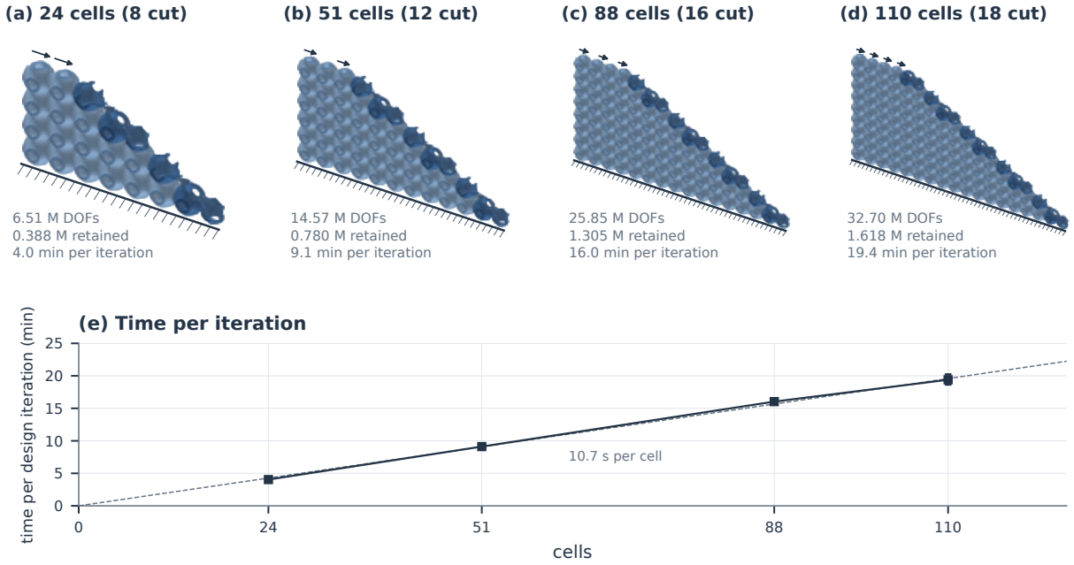
图 16: 规模算例中的板。(a-d) 胞元数为 24、51、88 和 110 的板，长宽比和切割方式与图 15 中的板相同，取均匀初始设计 \tau = 0.40 ，按同一比例绘制。各板立于其固支长边上（阴影线），对面施加沿长边方向的面内面力（箭头）。浅色为未切割胞元，深色为切割胞元。各子图注明切割有限元模型的自由度数、未约束的主自由度和每次设计迭代的平均用时。(e) 每次设计迭代用时随胞元数的变化（方块为平均值，误差棒为所计时迭代的范围）。虚线与胞元数成正比，对应平均每个胞元 10.7 s。内存占用见补充表 ST20。
