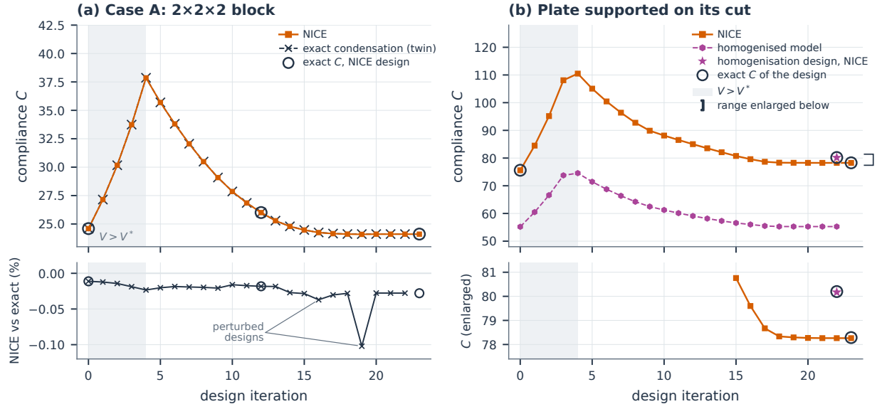
图 14: 基于 NICE 的厚度优化。(a) 算例 A: NICE 优化与采用精确静力凝聚的对照优化的柔度历程。空心圆为 NICE 设计在第 0、12 和 23 次迭代时的精确柔度。在体积由 1.25V^* 减小至 V^* 的过程中, 柔度先上升 (阴影, 第 0-3 次迭代)。下方条带: NICE 柔度相对于同一设计迭代处对照运行柔度的偏差 (线), 以及相对于同一设计精确柔度的偏差 (圆: -0.011\% 、 -0.018\% 、 -0.028\% )。两次运行的设计在第 0-4 次迭代时重合, 此后不同。在第 16 和 19 次迭代 (图中标注为 'perturbed designs'), NICE 设计曾被几何生成器的回退机制扰动 (补充表 ST19a)。(b) 切割面固支板。曲线为从均匀初始设计出发的 NICE 柔度, 以及均匀化宏观模型沿其自身优化路径的柔度 (虚线)。星号表示在切割几何上用 NICE 分析的均匀化设计, 位于最后一次宏观迭代处。空心圆为均匀初始设计、最终 NICE 设计和均匀化设计的精确柔度。阴影: V > V^* 的设计迭代。下方条带: 括号所标范围的放大, 自第 15 次迭代起。
