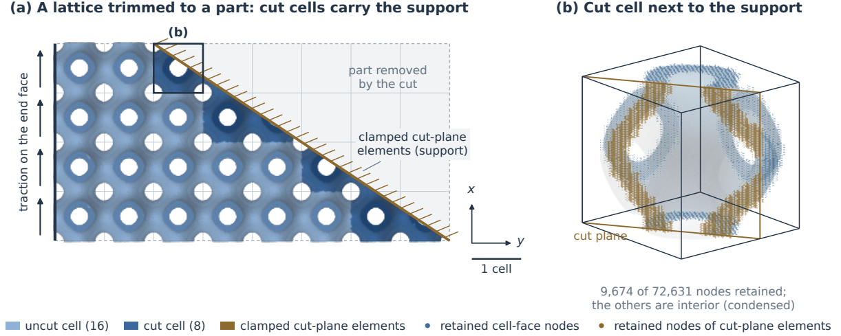
图 1: 按零件外形切割的点阵, 其切割胞元承担支撑。(a) 单层 8 \times 4 个 Schwarz-P 胞元 (式 (1), 均匀 \tau = 0.40 ) 经一个平面切割后的俯视图。该层含 16 个未切割胞元 (浅色) 和 8 个切割胞元 (深色); 被切去的部分以浅色虚线框绘出。板在切割处固支: 每个切割胞元中切割平面单元的全部自由度均被固定 (阴影线)。端面承受合力为单位值的面内面力载荷 (箭头)。(b) (a) 中框出的切割胞元, 壁面半透明, 并绘出切割平面。其 Q_2 模型共有 72,631 个节点, 其中位于胞元表面 (蓝色) 和切割平面单元中 (沙色) 的 9,674 个节点被保留。其余节点均为内部节点, 经静力凝聚消去。曲面由式 (1) 重构, 仅用于显示。
