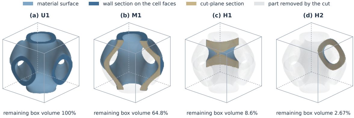
图 4: 代表性验证几何。(a) 未切割胞元 U1, (b) 中度切割胞元 M1, (c,d) 重度切割胞元 H1 和 H2, 各图采用相同的单位立方体尺度和观察方向。浅蓝色表示材料表面, 深蓝色表示胞元表面上的壁截面, 沙色表示切割平面上的截面。被切除的部分以半透明灰色绘出, 各胞元均从切割一侧观察。百分数为切割后剩余的立方体体积与单位立方体体积之比, 该体积未与薄壁材料求交。表面由式 (1) 在每轴 129 个点的网格上重构, 仅用于可视化。
