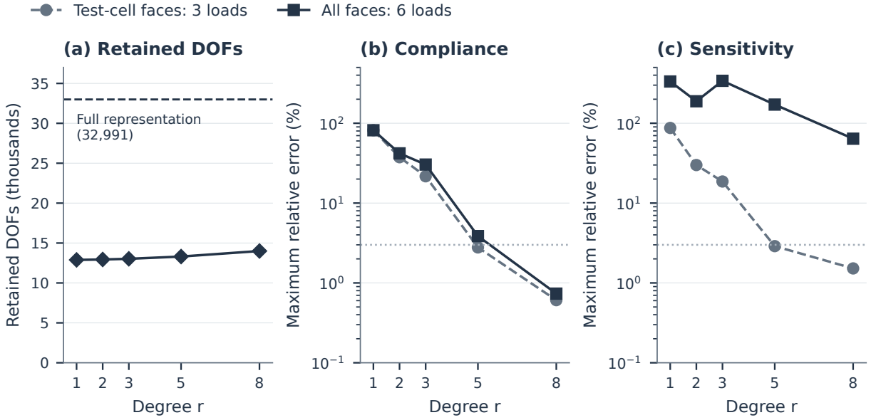
图 12: 限制胞元表面位移引起的响应误差。H1/x 的两个胞元均采用精确凝聚刚度矩阵, 并在每个胞元表面上采用 r 次 Bernstein 多项式。切割平面单元中不在胞元表面上的自由度不受限制。(a) 主自由度数目; 虚线表示完整表示的 32,991 个自由度。(b,c) 被测胞元表面三个载荷下或被测胞元与相邻胞元表面全部六个载荷下的最大柔度误差和最大被测胞元灵敏度误差。不计切割面上的面力载荷。误差以采用全部主自由度的解为基准, 水平线标示 3%。
