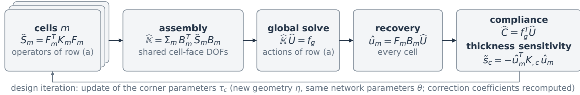
图 2: NICE 方法概览：单个胞元的凝聚刚度矩阵、装配与设计。(a) 网络预测内部位移之前，先从主自由度位移中分离出刚体运动部分，网络只处理其余的变形部分。随后叠加刚体位移场，并重新赋予给定的主自由度位移，得到 \hat{E}q 。两重网格修正 \mathcal{W} 在主自由度位移固定的条件下减小内部不平衡力，得到 \hat{u} = Fq 。依次施加胞元刚度矩阵 K 和转置 F^T ，即得主自由度上对应的节点力 \hat{S}q 。(a) 中的序关系 S \preceq \hat{S} \preceq \hat{S}_{\text{net}} 即命题 2 的结论，其中 \hat{S}_{\text{net}} 为未经修正的凝聚刚度矩阵。该序关系针对能量误差，不适用于灵敏度误差。(b) 各胞元的凝聚刚度矩阵在共享的胞元表面自由度上装配，随后求解装配系统。由装配解恢复每个胞元的位移，并计算柔度和厚度灵敏度。每次设计迭代更新角点厚度参数，因而改变每个胞元的几何。网络参数保持不变， \mathcal{W} 的系数则重新计算。
