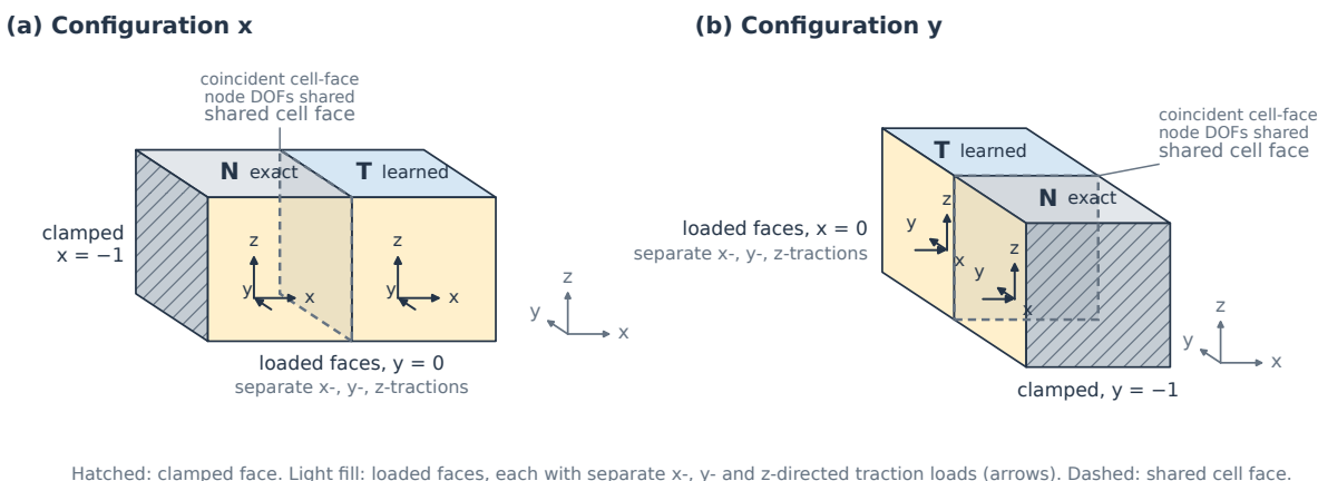
图 9: 两胞元装配的支撑与载荷。(a) 构型 x : 相邻胞元平移 (-1, 0, 0) ，面 x = -1 固支，面力载荷作用于 y = 0 处的表面。(b) 构型 y : 平移量为 (0, -1, 0) ，面 y = -1 固支，面力载荷作用于 x = 0 处的表面。被测胞元 (T) 和相邻胞元 (N) 的加载面上分别施加 x 、 y 、 z 方向的面力载荷。重合的胞元表面节点自由度在界面上共享；切割平面单元中不在胞元表面上的自由度只属于所在胞元。切割的被测胞元还承受切割面上的三个面力载荷，这些载荷单独分析。
