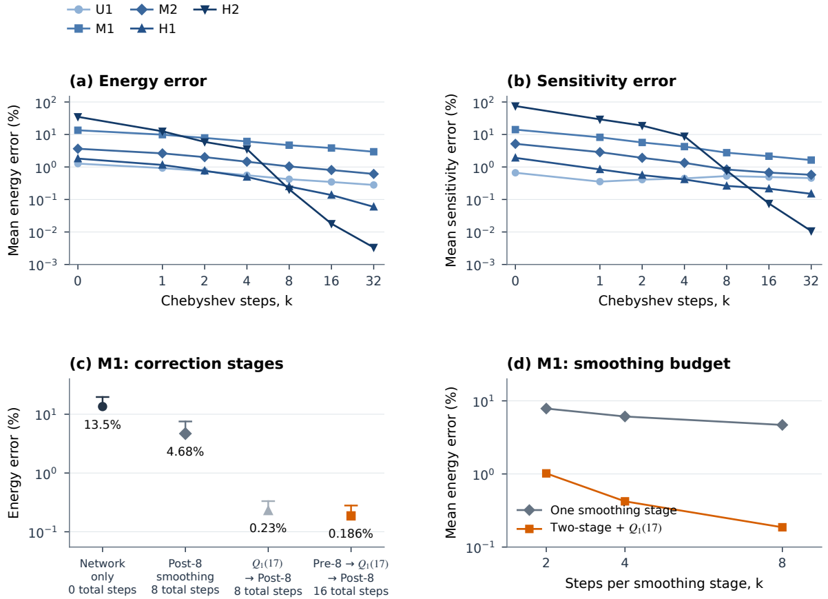
图 8: 固定网络参数下对基础网络的修正。(a,b) 五个胞元在 Chebyshev 光滑过程中的平均能量误差与灵敏度误差。(c) M1 在四种情形下的结果: 无修正; 八步光滑; 粗网格校正后接八步光滑; 粗网格校正前后各八步光滑。圆点表示均值, 端帽表示第 90 百分位数。(d) M1 的平均能量误差随每个光滑阶段步数 k 的变化, 分别对应单独一个光滑阶段, 以及由 k 步前光滑、 Q_1(17) 粗网格校正和 k 步后光滑组成的循环。所有子图均采用面力载荷、固定的主自由度位移和 a = b/30 。(a,b) 中步数轴在零到一之间为线性刻度, 此后为对数刻度。
