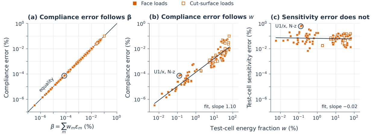
图 11: 柔度误差随被测胞元的应变能占比减小, 灵敏度误差则不随之减小。NICE 在七个被测胞元的十四种构型中的结果, 每个点对应一个载荷, 共有 84 个面载荷 (实心标记) 和 30 个切割面载荷 (空心标记)。各载荷上的最大值见补充表 ST08 和补充表 ST09。(a) 柔度误差与 \beta = \sum_m w_m \varepsilon_m 的关系, 其中应变能占比 w_m = q_m^T S_m q_m / C 和能量误差 \varepsilon_m = q_m^T (\hat{S}_m - S_m) q_m / (q_m^T S_m q_m) 均在精确装配的主自由度位移处计算。只有学习的被测胞元对 \beta 有贡献。直线表示二者相等。对每个载荷, 柔度误差均为 \beta 的 0.963 至 1.004 倍。比值高于 1 的五个载荷, 其超出量至多为柔度的 7.8 \times 10^{-10} , 而胞元对求解的残差功可达柔度的 1.8 \times 10^{-8} (补充说明 S4.3)。(b) 柔度误差和 (c) 被测胞元灵敏度误差随被测胞元精确应变能占比 w 的变化; 实线为对数坐标下的最小二乘拟合。圈出的点为 U1/x 在相邻胞元表面 z 向面力载荷下的结果。其余变体的相应结果见图 S04。
