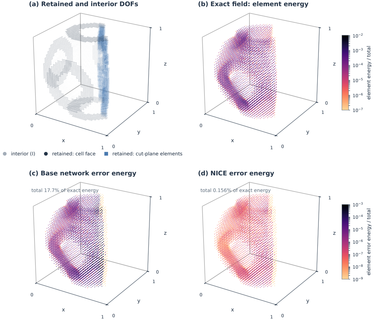
图 7: M1 的主自由度及内部位移误差的空间分布。(a) 胞元表面上的主自由度、切割平面单元的主自由度和内部自由度。(b) 一个面力载荷测试位移下精确位移场的体单元能量，以其总能量归一化。(c,d) 在相同主自由度位移下，基础网络与 NICE 误差的体单元能量，以 (b) 中精确位移场的总能量归一化，采用统一色标。切割平面单元的自由度均为主自由度，因而不含误差。
