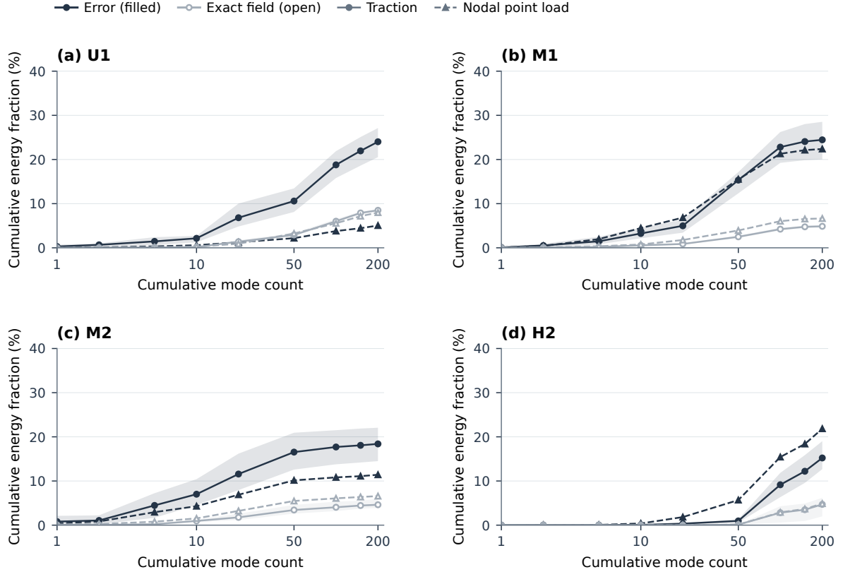
图 6: 基础网络内部位移误差的谱分布。各子图依次为 U1、M1、M2 和 H2。模态满足 Av = \lambda Dv ，其中 D = \text{diag}(A) ，并按特征值递增排序。深色实心标记表示误差，浅灰色空心标记表示精确内部位移场。带圆形标记的实线对应面力载荷，带三角形标记的虚线对应集中节点载荷。曲线为各测试位移的均值。色带为面力载荷下各测试位移的第 10 至第 90 百分位数。每条累积占比曲线均以其自身位移场或误差的内部总能量归一化。
