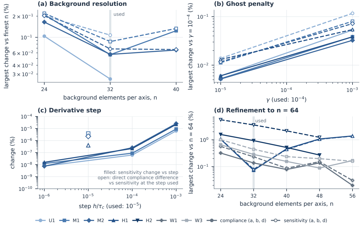
图 S01: CutFEM 参考解的验证 。单个胞元在一个胞元表面上固支，并在另一个面上沿三个笛卡尔坐标方向分别受单位面力载荷作用。在 (a)、(b) 和 (d) 中，带实心标记的实线表示柔度，带空心标记的虚线表示厚度灵敏度，均取三个载荷下的最大相对变化。(a) 相对于所计算的最细背景分辨率的变化，U1 为 n = 40 ，M1 和 M2 为 n = 48 ；全文所用参考解取 n = 32 。(b) ghost 罚项系数偏离全文所用值 10^{-4} 时的变化。(c) 实心：矩导数的有限差分步长偏离全文所用值 h_c = 10^{-5}\tau_c 时灵敏度的最大相对变化，在 10^{-3}\tau_c 处至多为 2.6 \times 10^{-5}\% ，在 10^{-4}\tau_c 处再小一百倍；空心：在所用步长下，柔度中心差分与灵敏度之间的最大相对差异。(d) H1、H2 以及 NICE 误差最大 (W1) 和壁厚最薄 (W3) 的验证胞元加密至 n = 64 ，数据见表 ST10；H2 没有 n = 56 的解。
