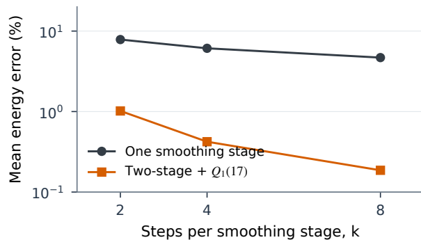
(d) M1: smoothing budget
