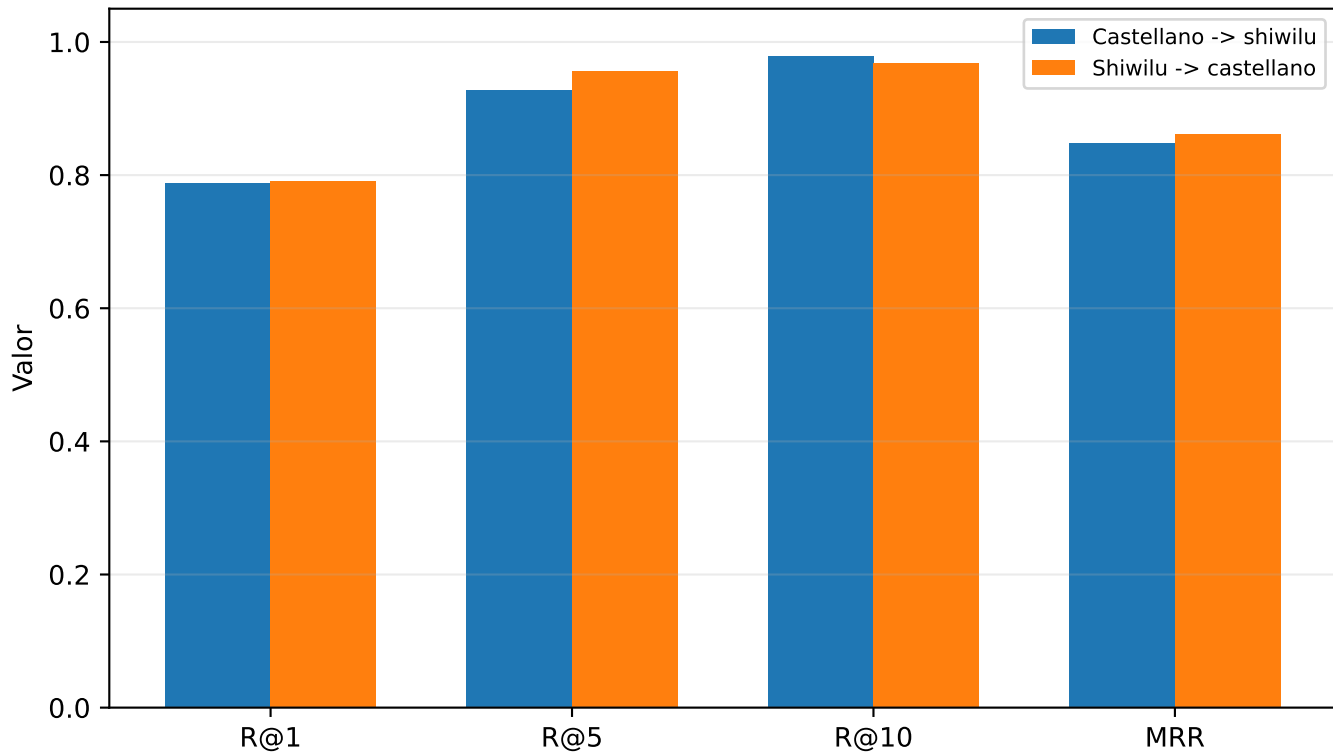
Metricas finales del modelo v3
