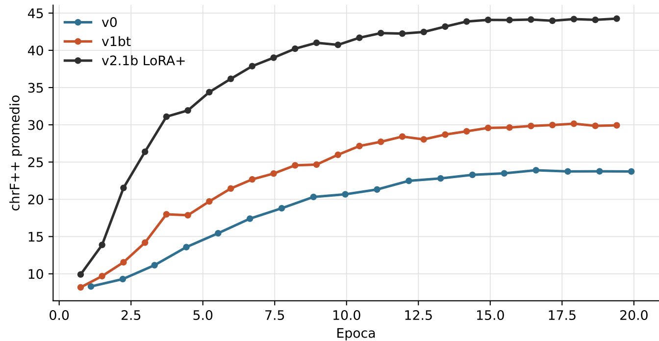
chrF++ de validación durante el entrenamiento
