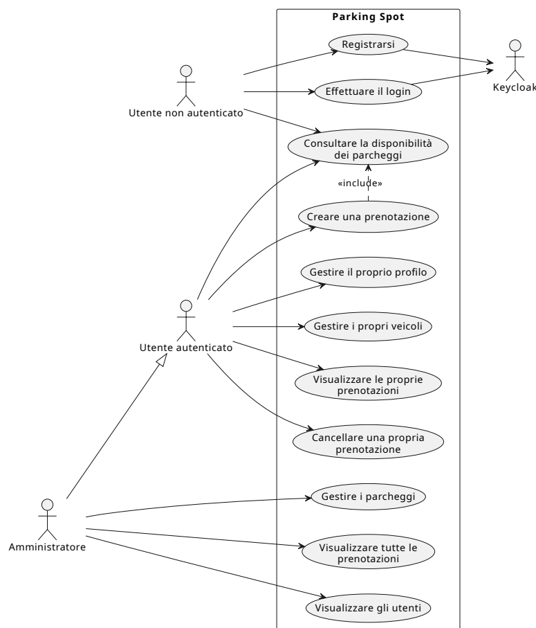
Figura 1: Diagramma UML dei casi d'uso dell'applicazione.
