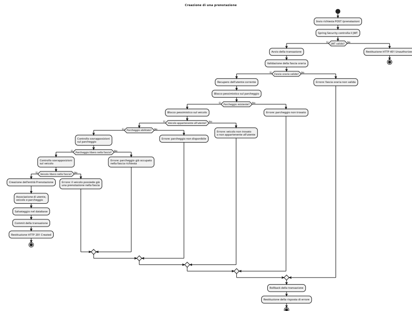
Figura 2: Activity Diagram UML della creazione di una prenotazione.
