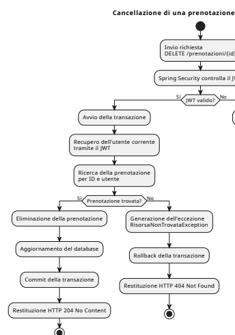
Figura 3: Activity Diagram UML della cancellazione di una prenotazione.
