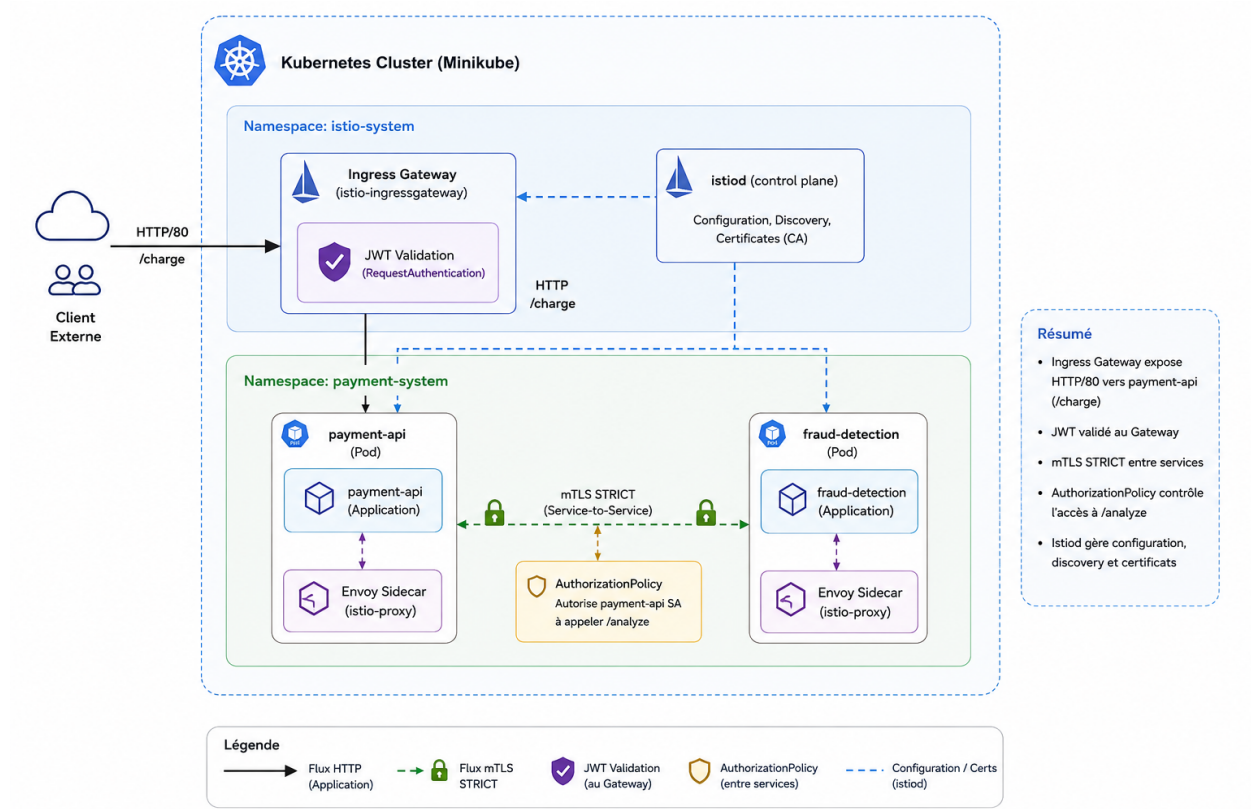
Figure 2.1 — Architecture du prototype Service Mesh — Kubernetes/Minikube avec Istio
