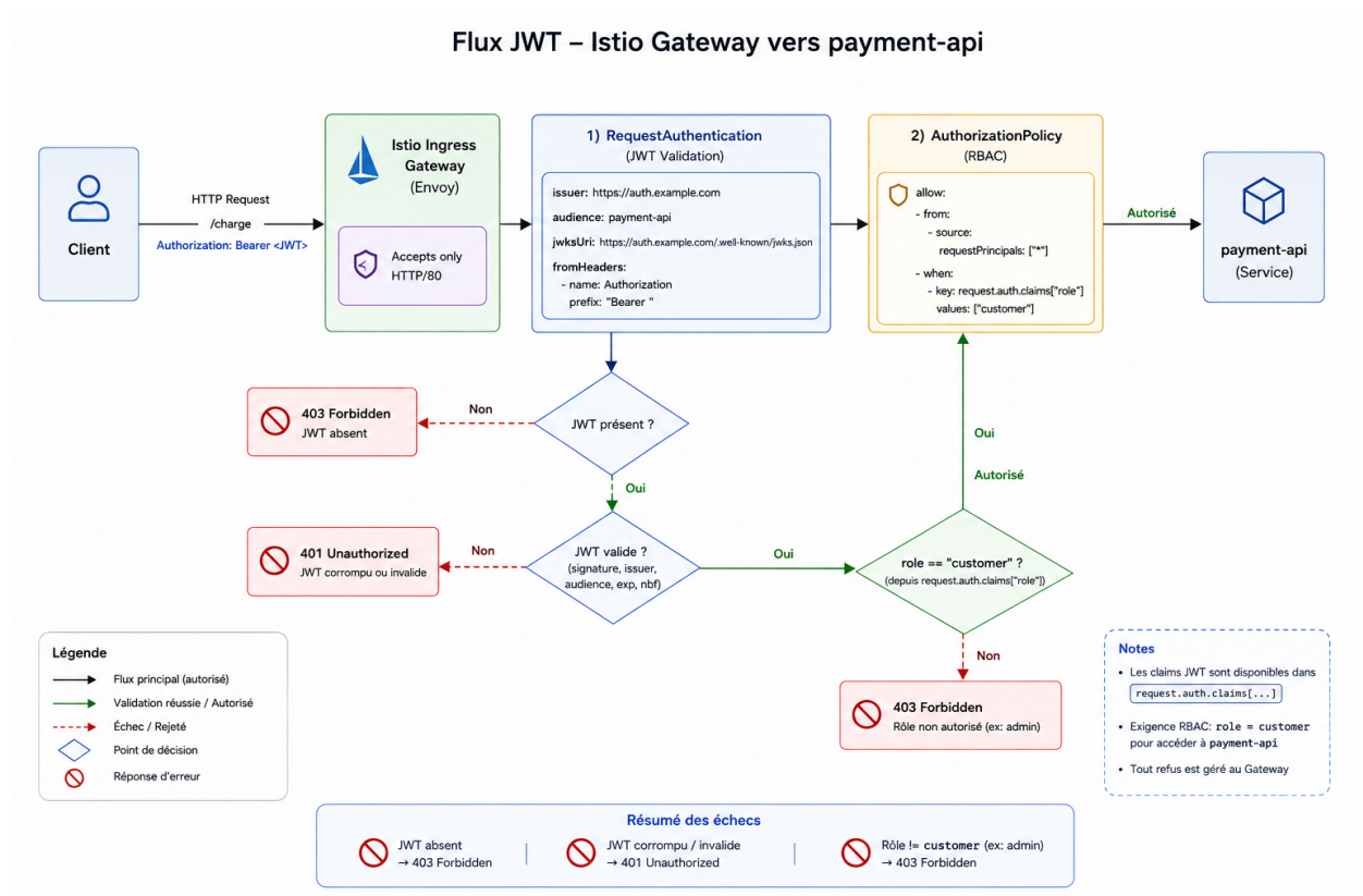
Figure 4.9 — Figure 4.X — Flux JWT : validation par RequestAuthentication et contrôle d'accès par AuthorizationPolicy au niveau de l'Istio Ingress Gateway.
