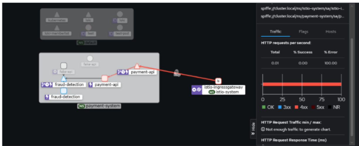
Figure 4.9 — Test T5 — envoi d'un JWT à signature corrompue, rejet HTTP 401 et trafic en erreur visible dans Kiali
