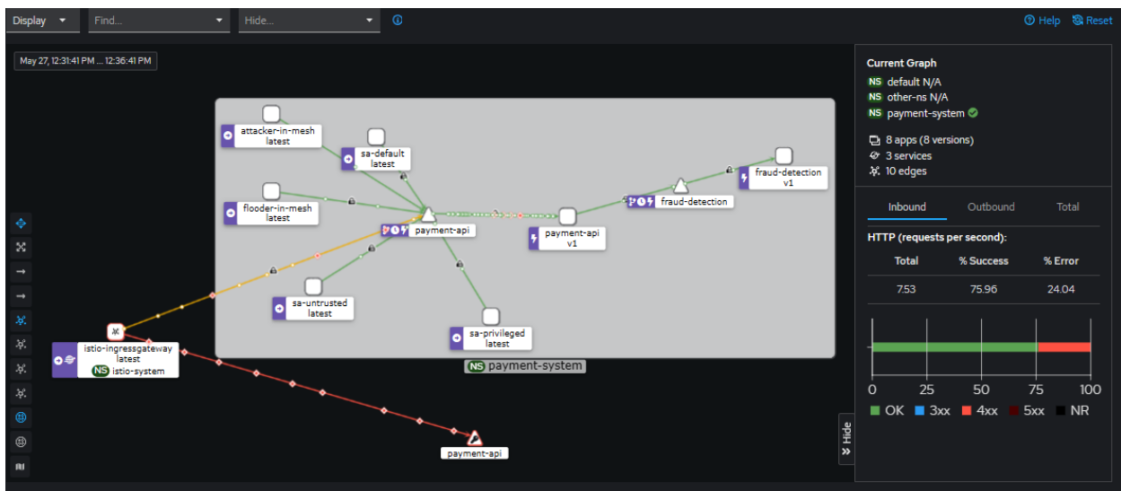
Figure 4.13 — Kiali — Même topologie pendant une phase d'attaque plus intense. Le taux d'erreur global monte à 24,04 % : les arêtes passent de vert à orange puis rouge selon l'intensité des rejets. Le lien istio-ingressgateway → payment-api est entièrement rouge, confirmant que les requêtes du flooder-outside (sans JWT valide ou dépassant le rate limit) sont massivement rejetées.
