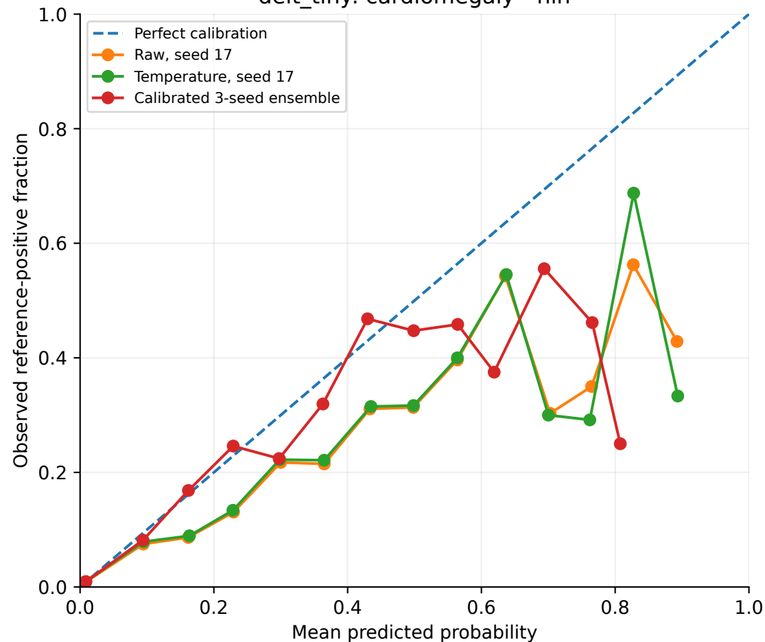
deit_tiny: cardiomegaly - nih
