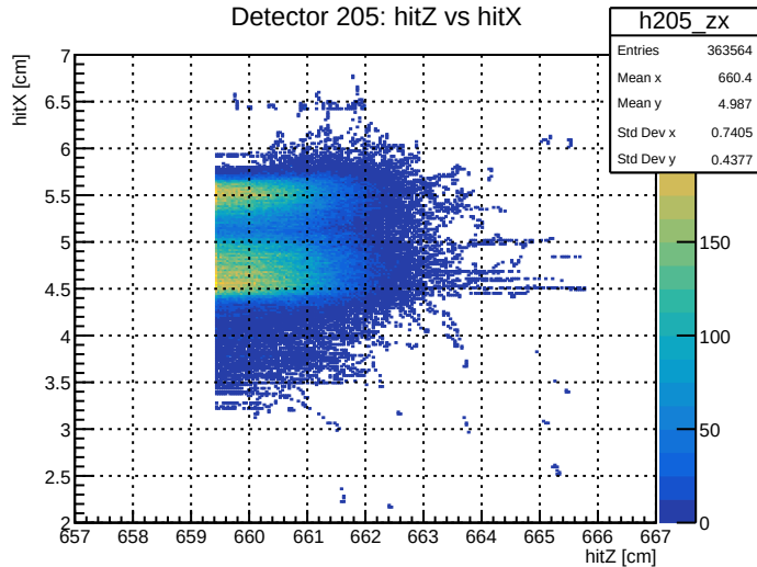
Detector 205: hitZ vs hitX
