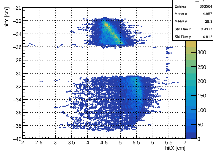
Detector 205: hitX vs hitY
