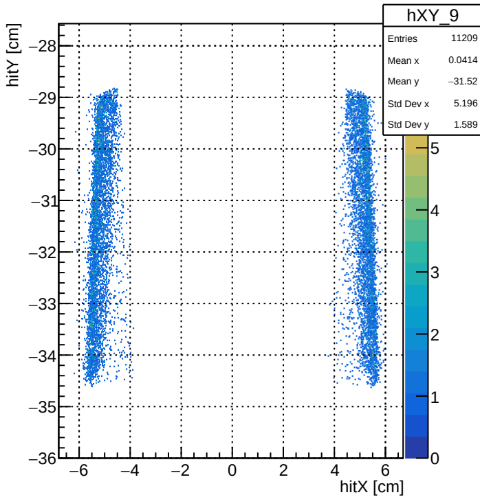
hitX vs hitY - Detector 9: Moller Detector
