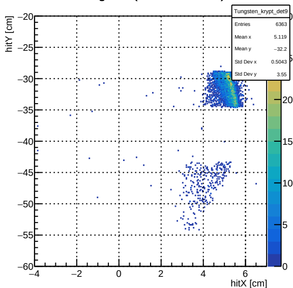
Tungsten (Mask Interacts)
