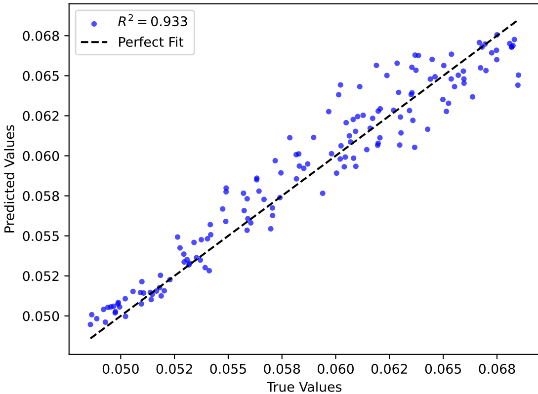
Predicted vs. Actual Values (Laplace)
