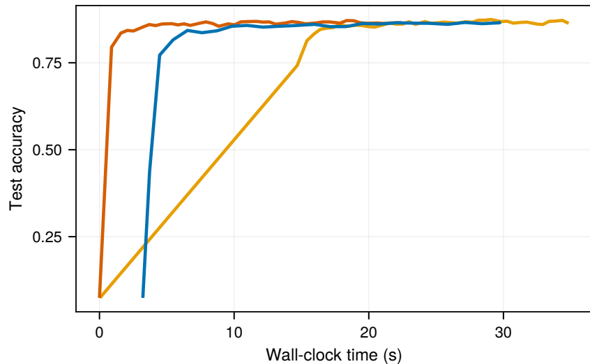
(d) Test accuracy vs. time
