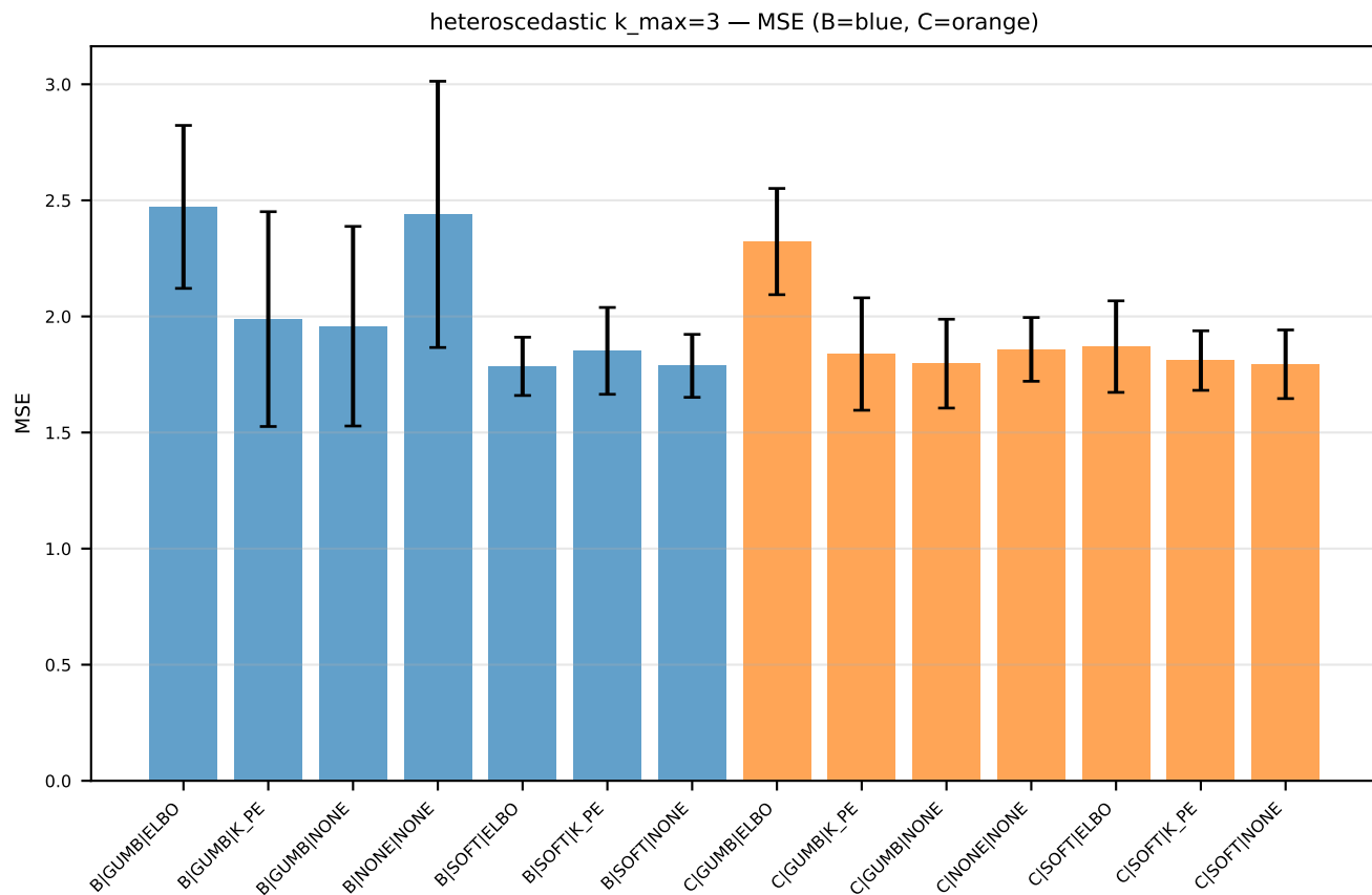
heteroscedastic k_max=3
