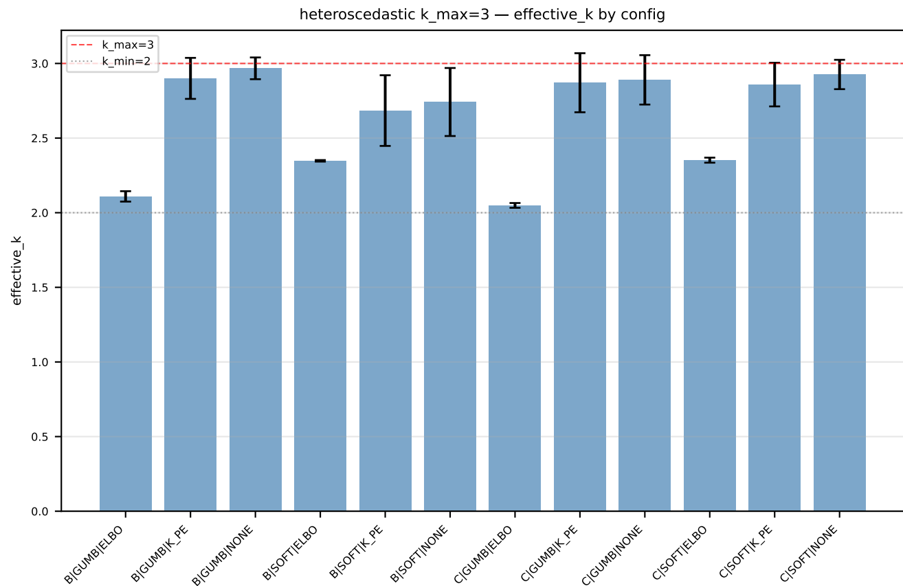
heteroscedastic k_max=3
