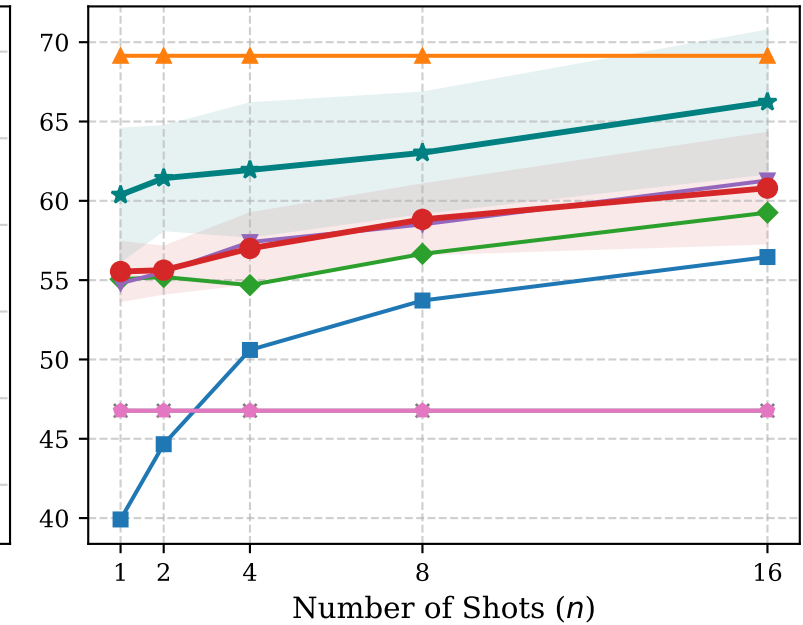
(d) Resisc45 Water
