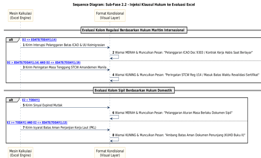
Gambar 23 DS, Pembuatan Logika Excel dengan Terapan Hukum Berlaku
