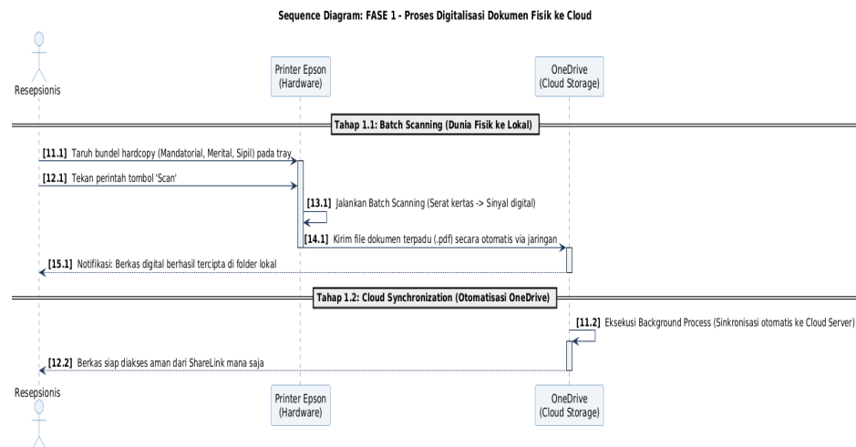
Gambar 20 Diagram Sequences Digitalisasi Doc. Pelaut
