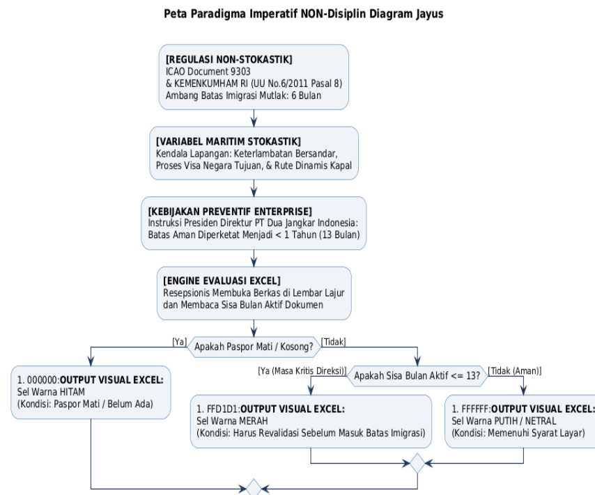
Gambar 26 Keputusan-2 Passport Kondisi berdasarkan Case Negara Bendera & MRZ ICAO
