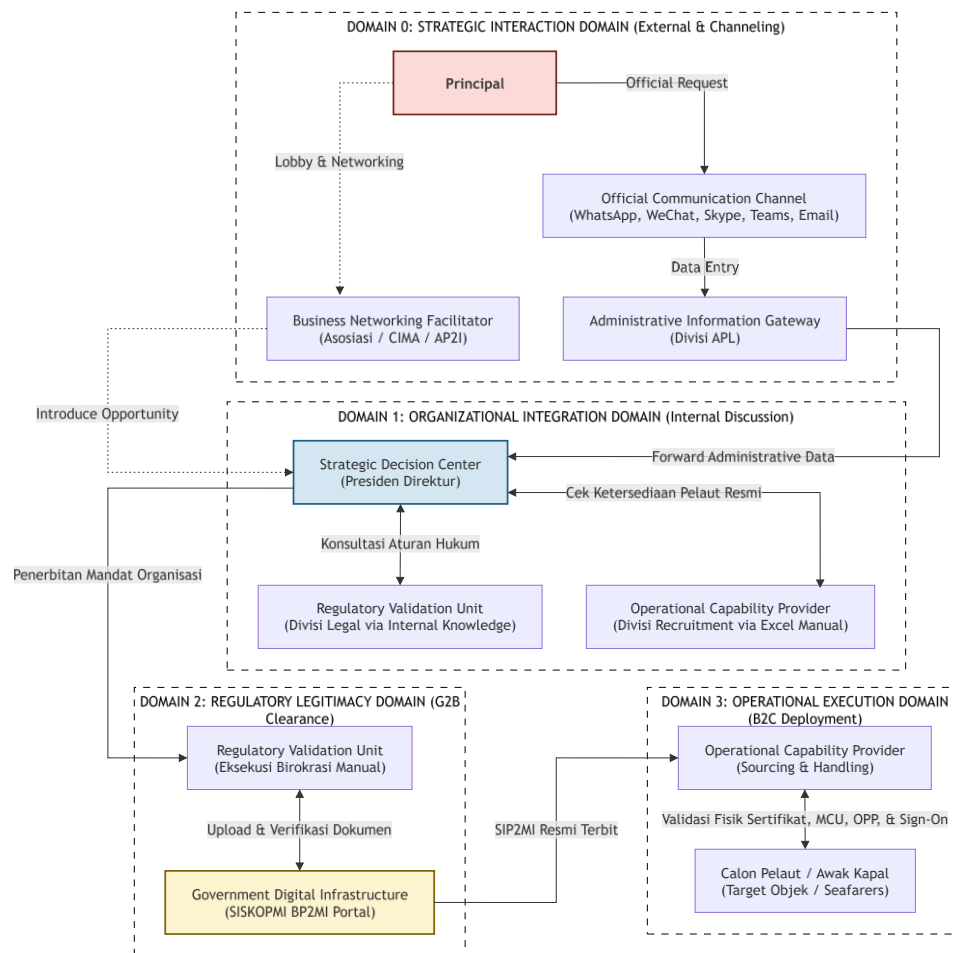
Gambar 6 Abstrak Pemodelan Alur Pembukaan Vacancy
