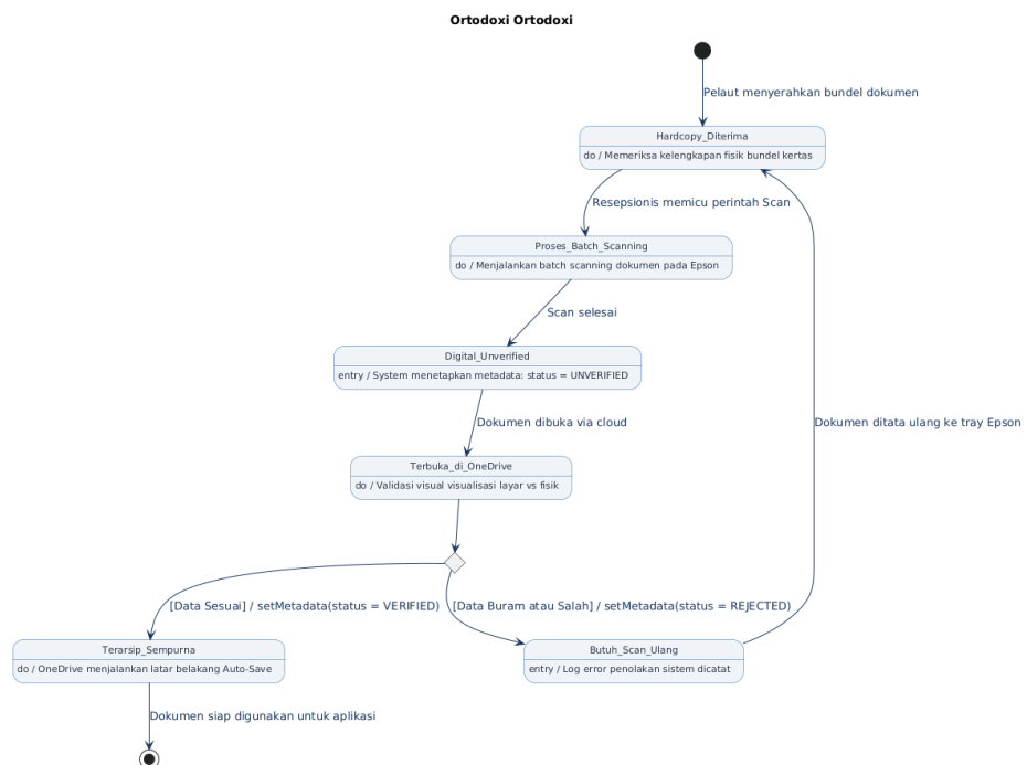
Gambar 18 Tahap Scanning State Machine yang dihadapi resepsionis
