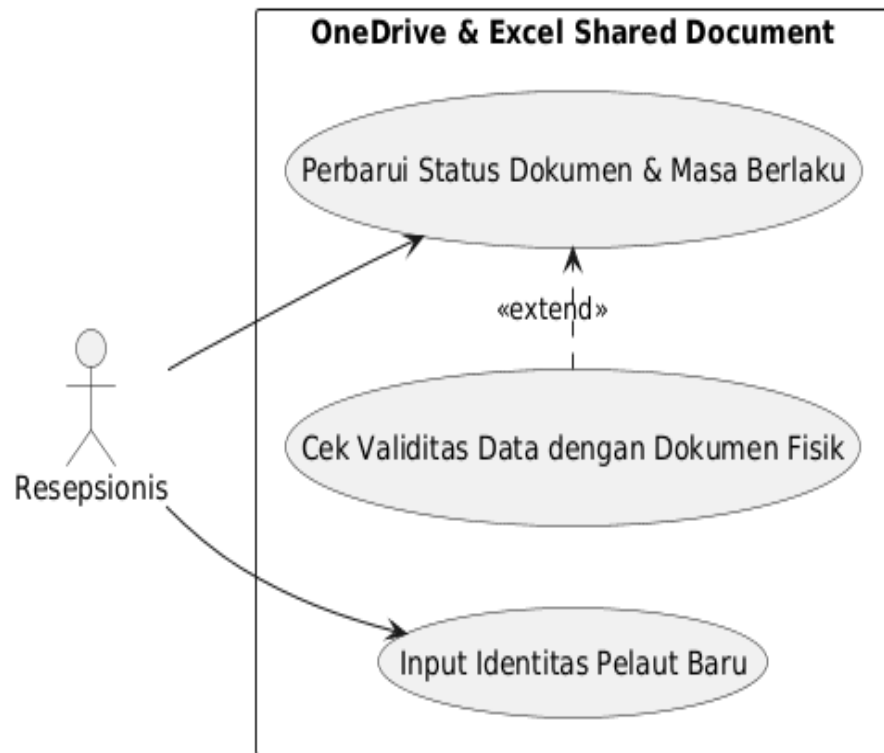
Gambar 21 Use Case, Sesuai Peta Realitas Kantor
