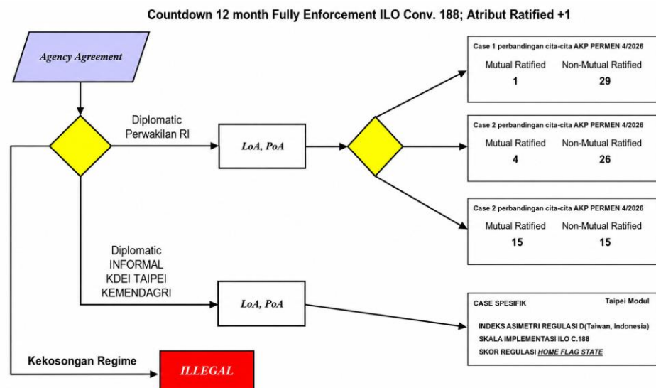
Gambar 7 Peta Stokastis 30 ratified konvensi kemaritiman, Indonesia
