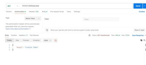
Gambar 2.2 Invalid Token
