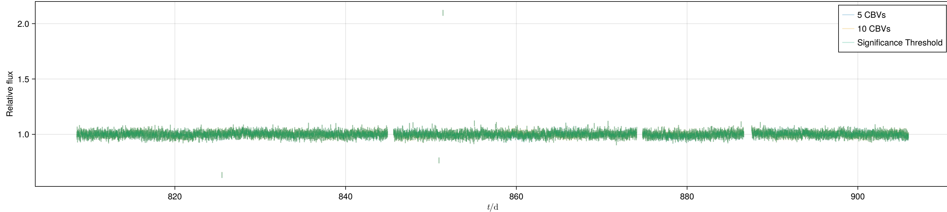
hlsp_iris_kepler_kepler_kplr002570350-q09_kepler_v1.0_lc_detrended.fits
