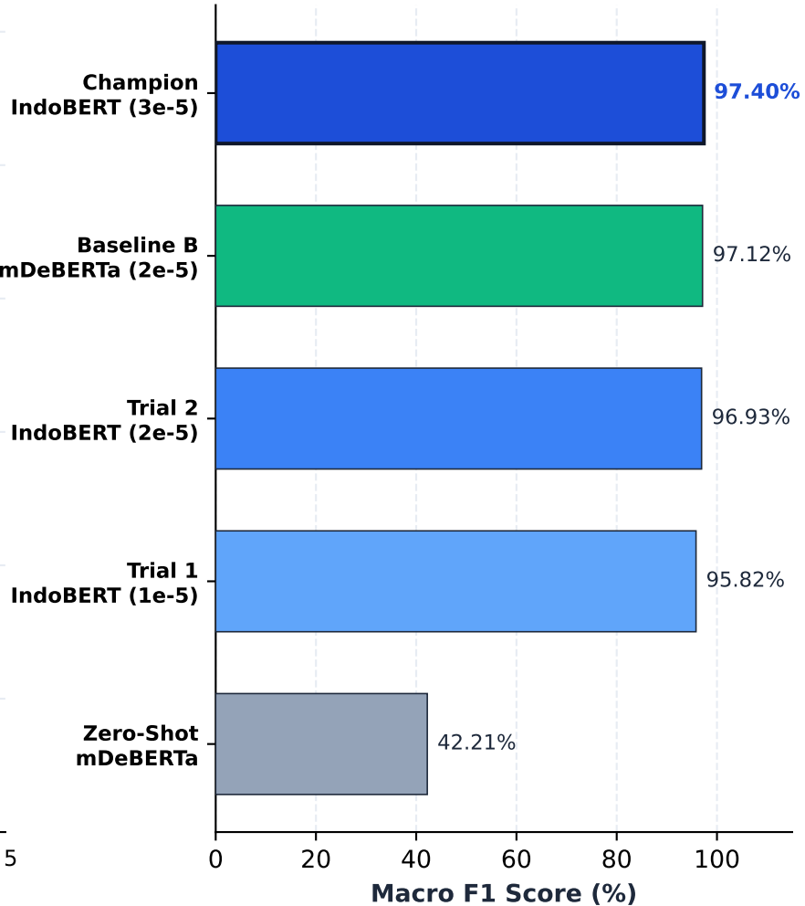
(c) Held-Out Macro F1 Benchmark
