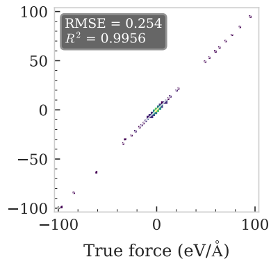
LRT Het.
