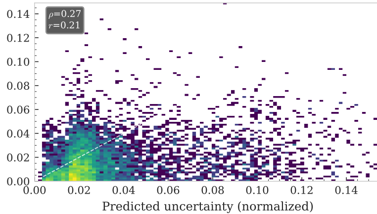
LRT
