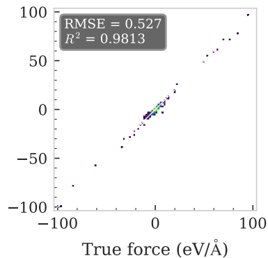
LRT
