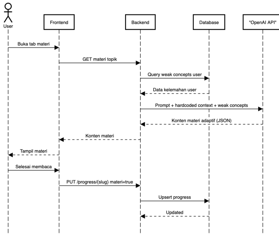
Gambar IV.5 Sequence Diagram FT-04 Tampilkan Materi, FT-10 Generate LLM, dan FT-14 Adaptasi Konten
