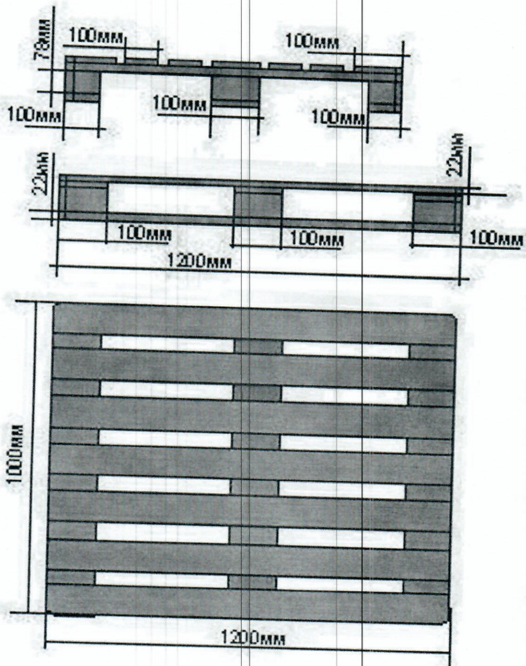
Рисунок 1.- Поддон деревянный 1200*1000*144 мм однонастильный четырехзаходный бывший в употреблении
