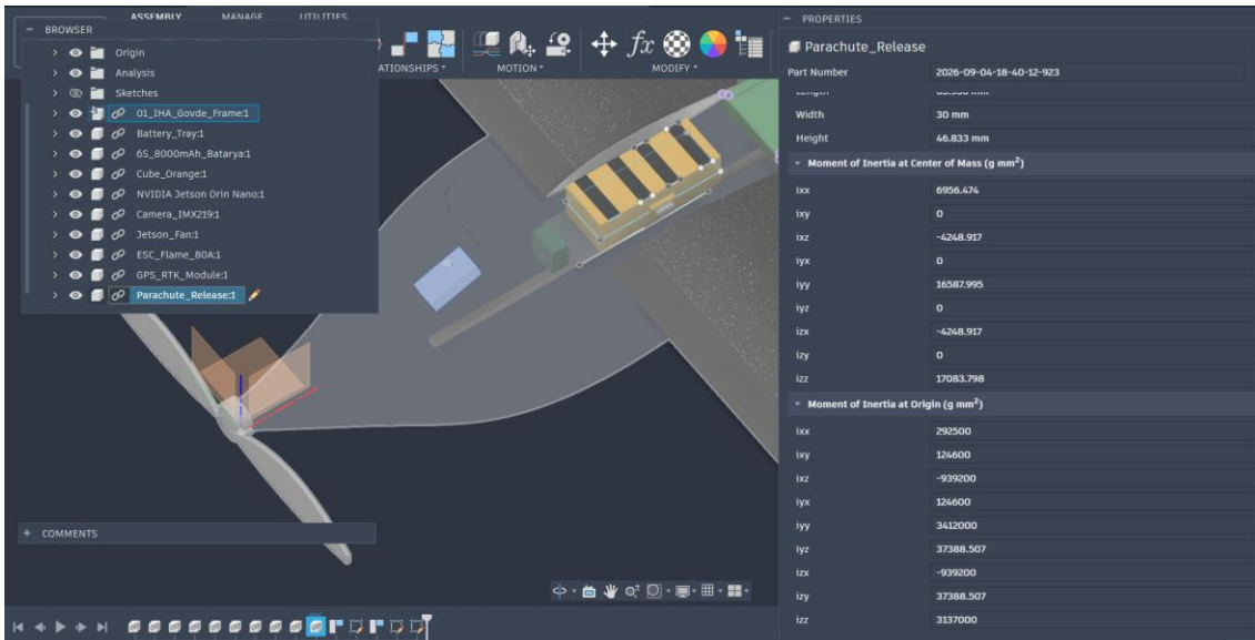
Şekil 3.1.2.31. Paraşüt bırakma mekanizmasının ikinci görünüşü. Tetikleme strokunun kapak ve gövde ile çakışmaması doğrulanmalıdır.
